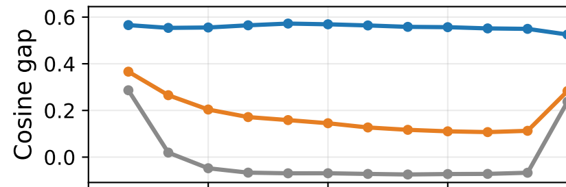
LaTa
