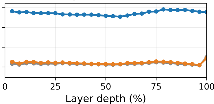
Qwen3-0.6B
