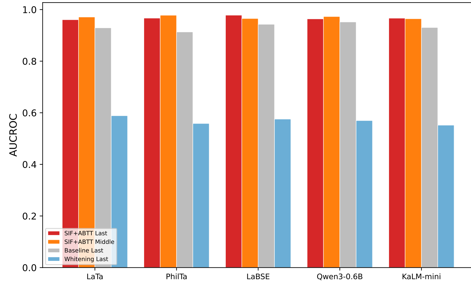
(A) AUCROC
