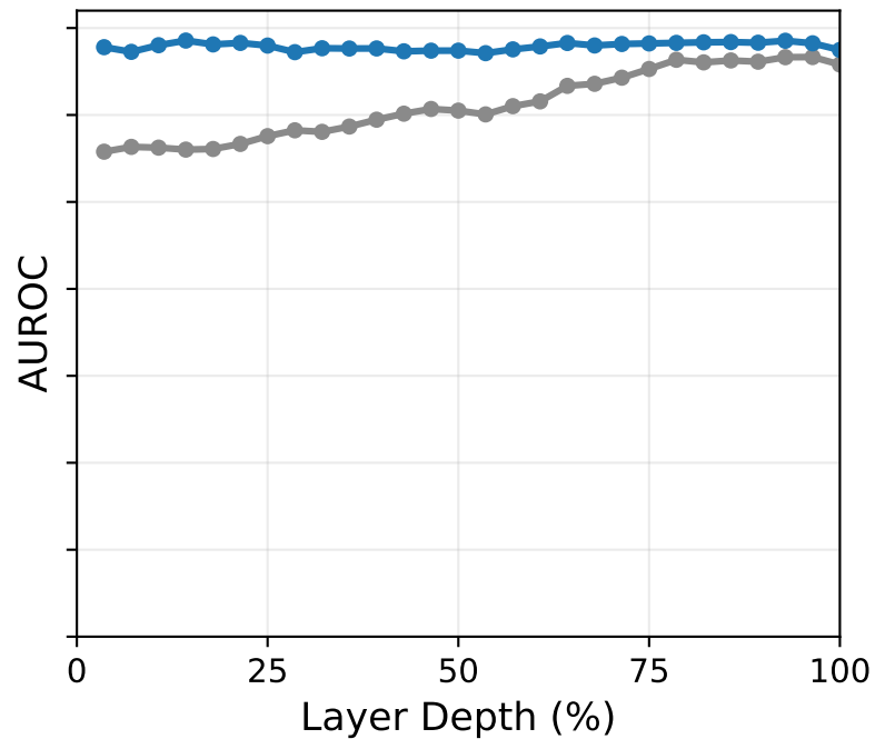
Qwen3-0.6B
