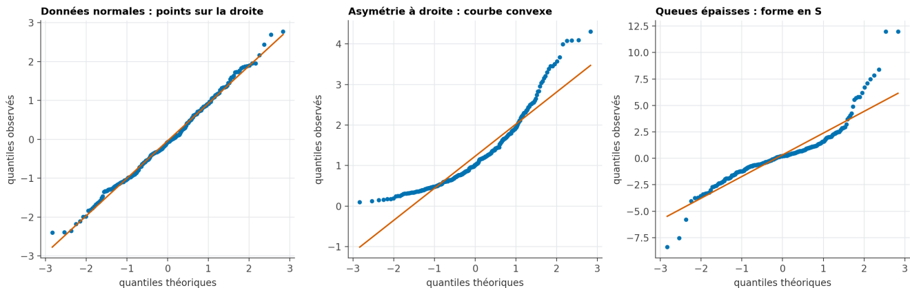
FIGURE 11 – Trois signatures caractéristiques sur un diagramme quantile-quantile
