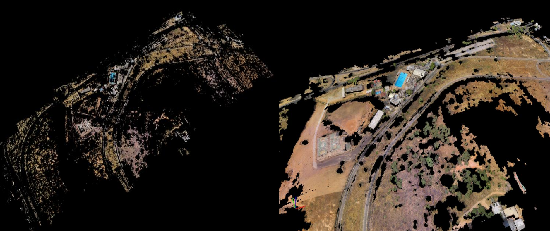
FIGURA 4. Nube de puntos, reconstrucción 3D de la superficie
