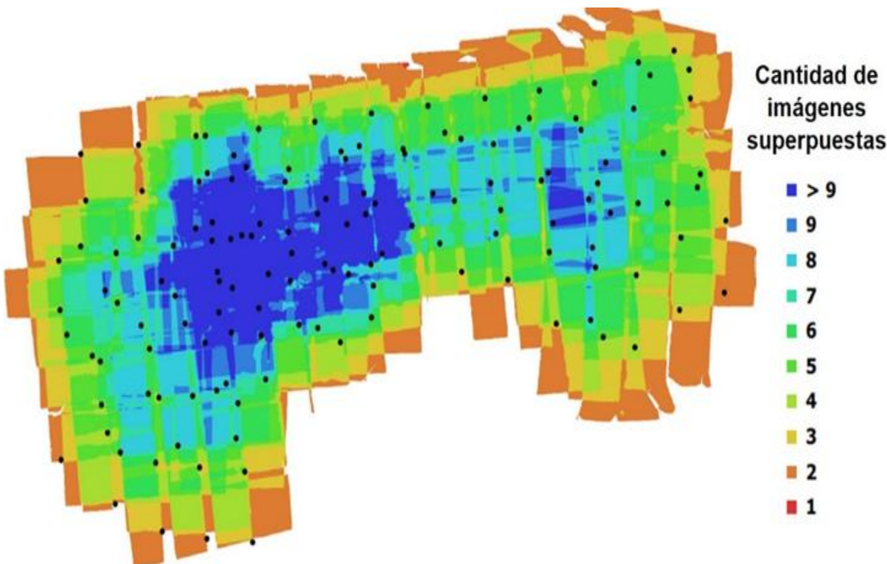
FIGURA 6. Posición de puntos de enlace y solapamiento entre imágenes.
