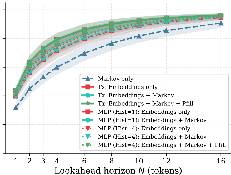
Precision@16
