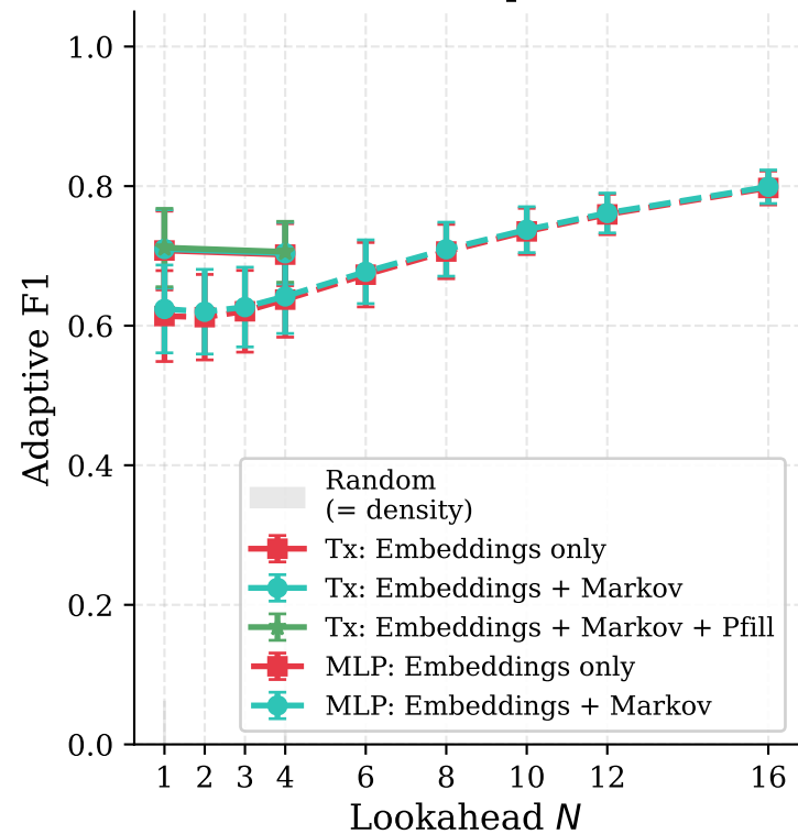
(a) Raw Adaptive F1
