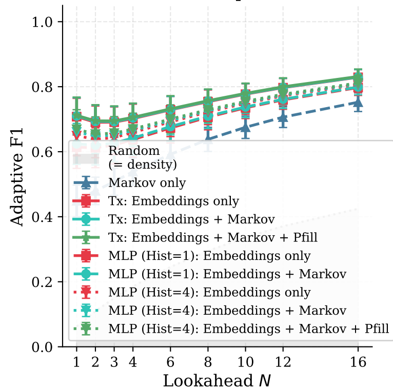
(a) Raw Adaptive F1
