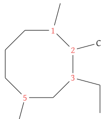
(b) 2-Chloro-3-ethyl-1,5-dimethyl-cyclooctane
