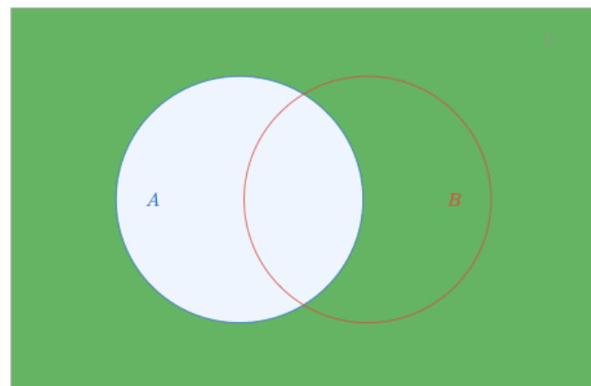
\bar{A}
