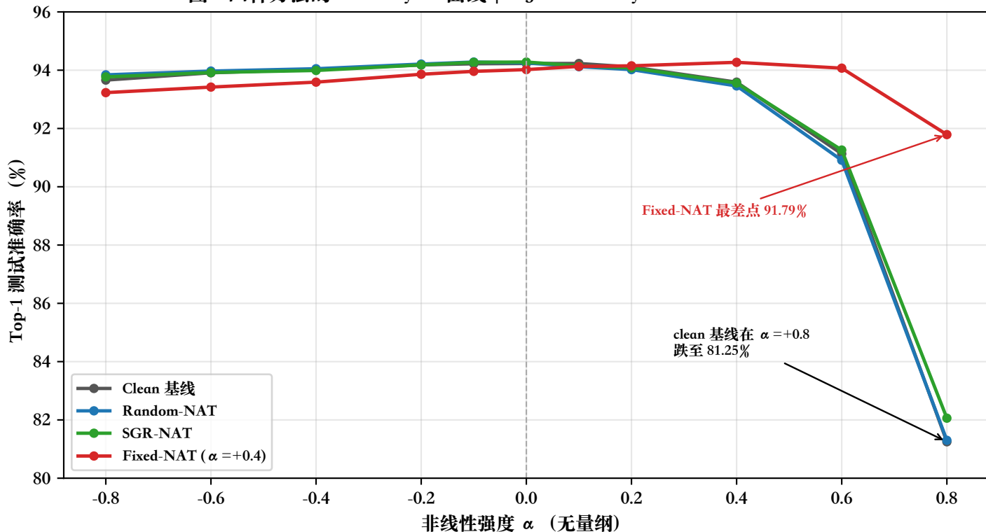
图3 四种方法的 Accuracy- \alpha 曲线 | Fig. 3 Accuracy- \alpha curves of four methods
