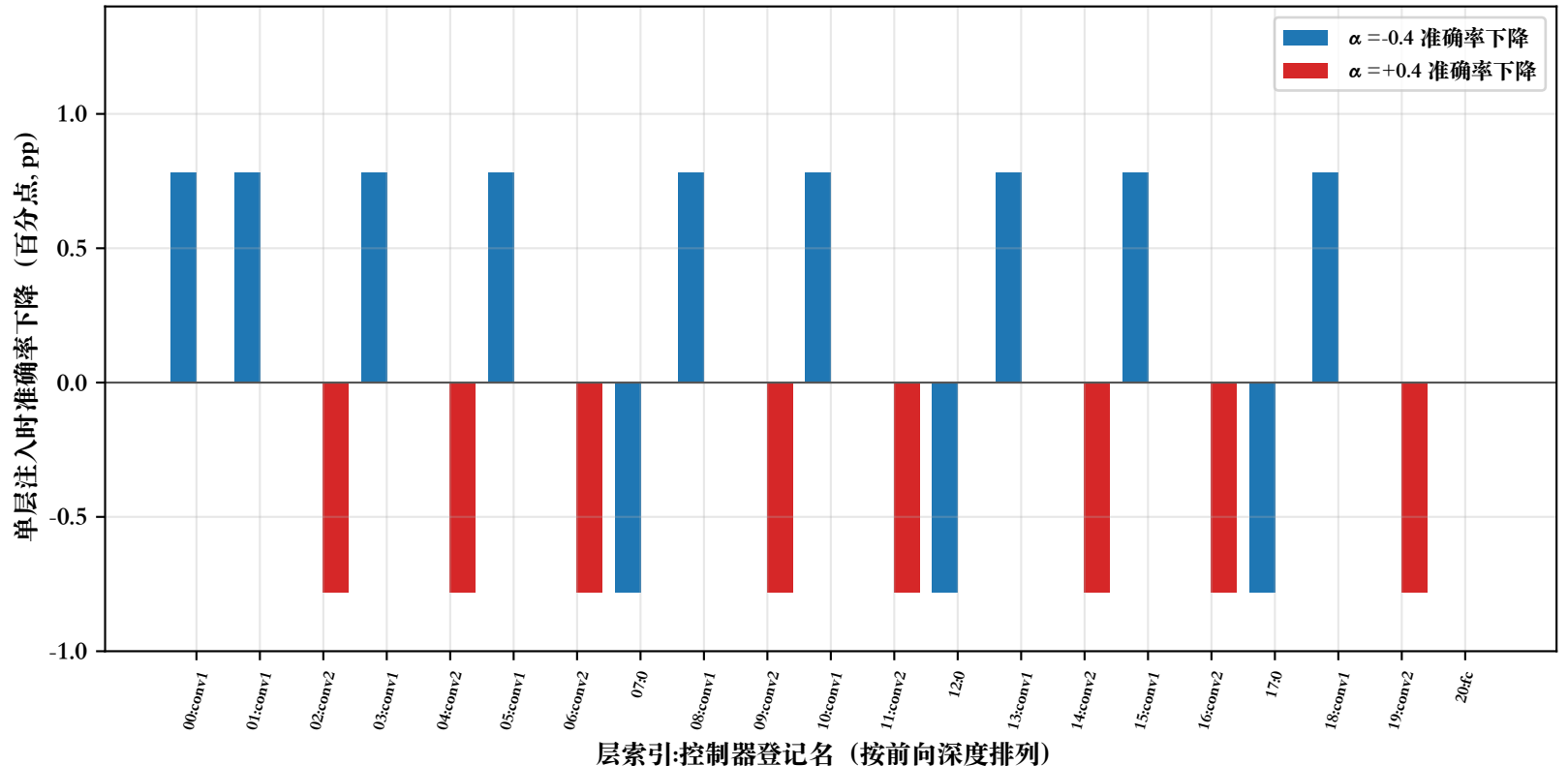
图4 单层注入敏感性 (128 样本批, 分辨率 0.78 pp) | Fig. 4 Per-layer sensitivity
