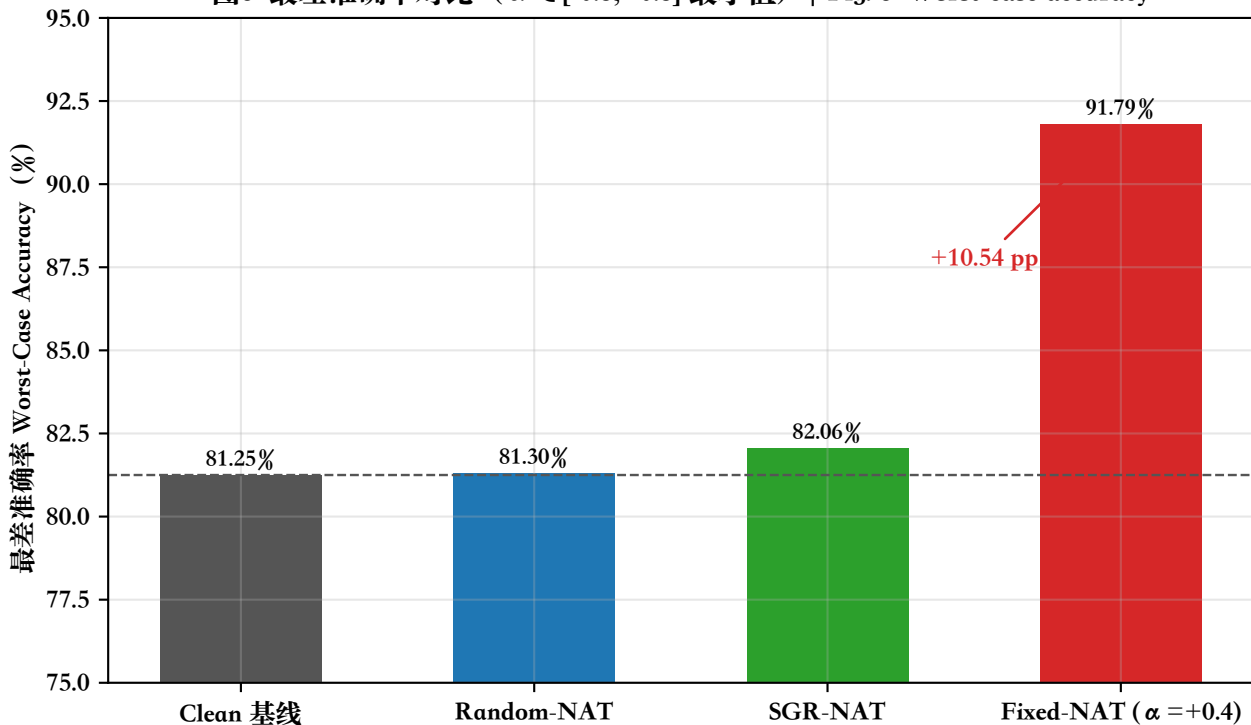
图6 最差准确率对比 ( \alpha \in [-0.8, +0.8] 最小值) | Fig. 6 Worst-case accuracy
