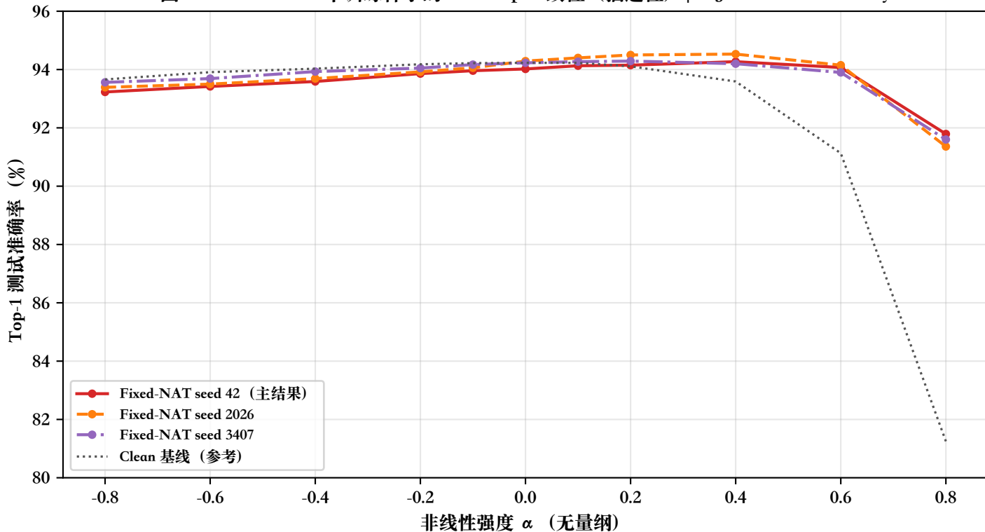
图10 Fixed-NAT 三个训练种子的 \alpha -Sweep 一致性 (描述性) | Fig. 10 Seed consistency
