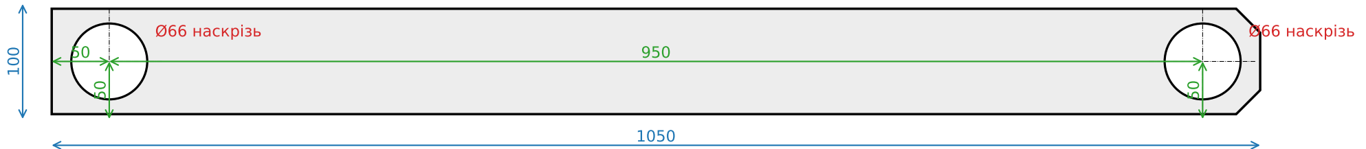
Права стінка
