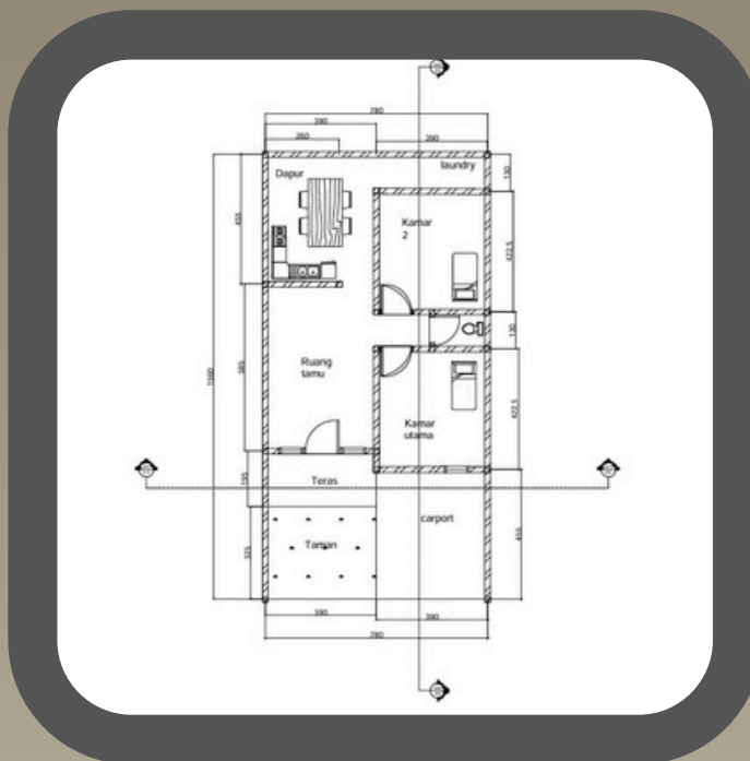
DENAH RUMAH TYPE 36
