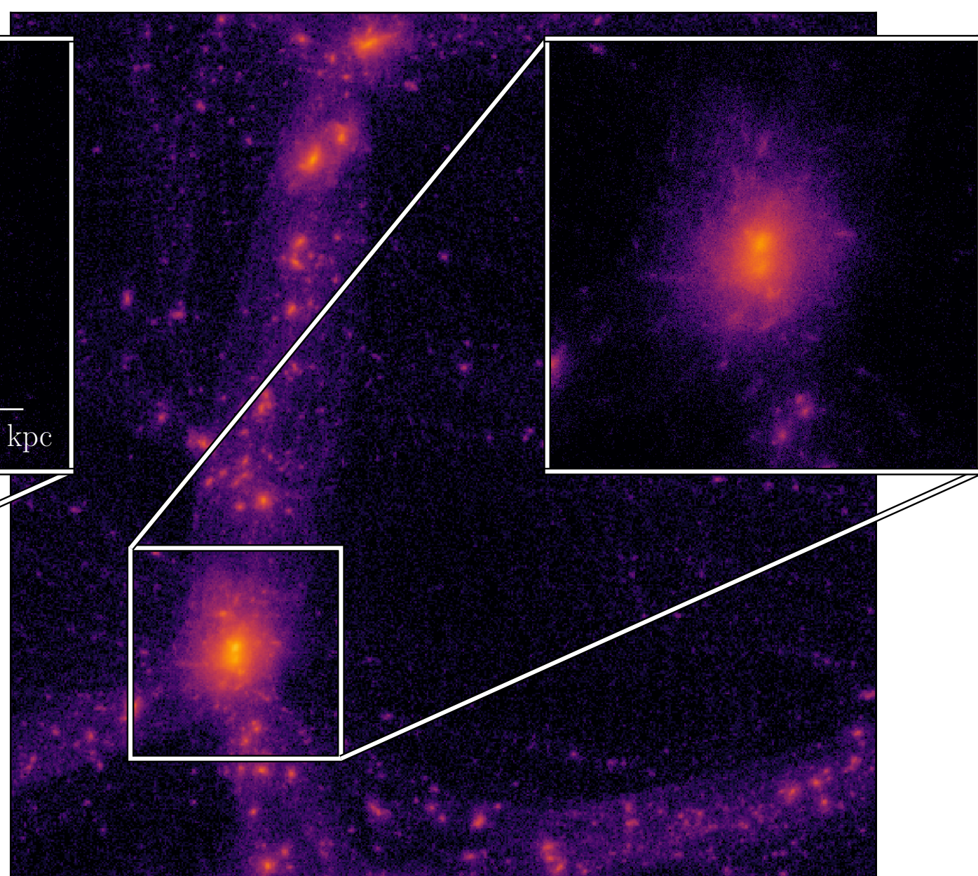
COLA
