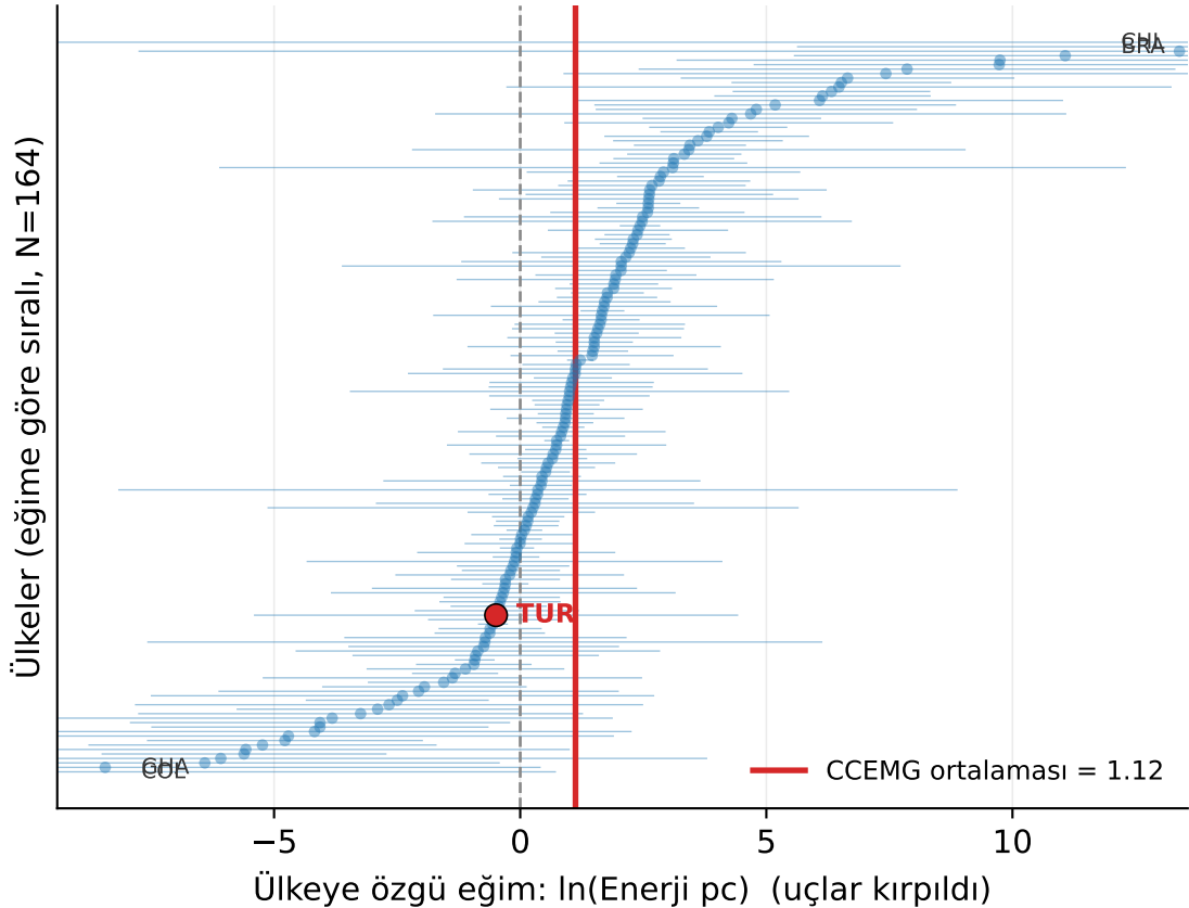
Şekil 3. CCEMG ülke-bazlı eğim heterojenliği
