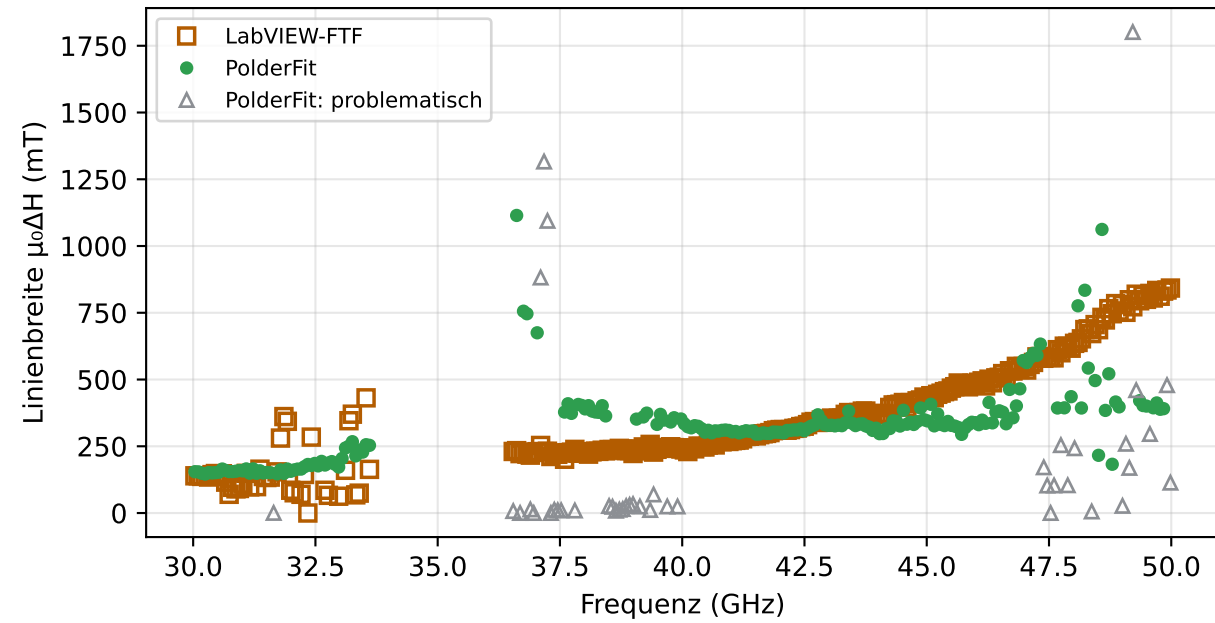
Differenz Linienbreite je Frequenz
