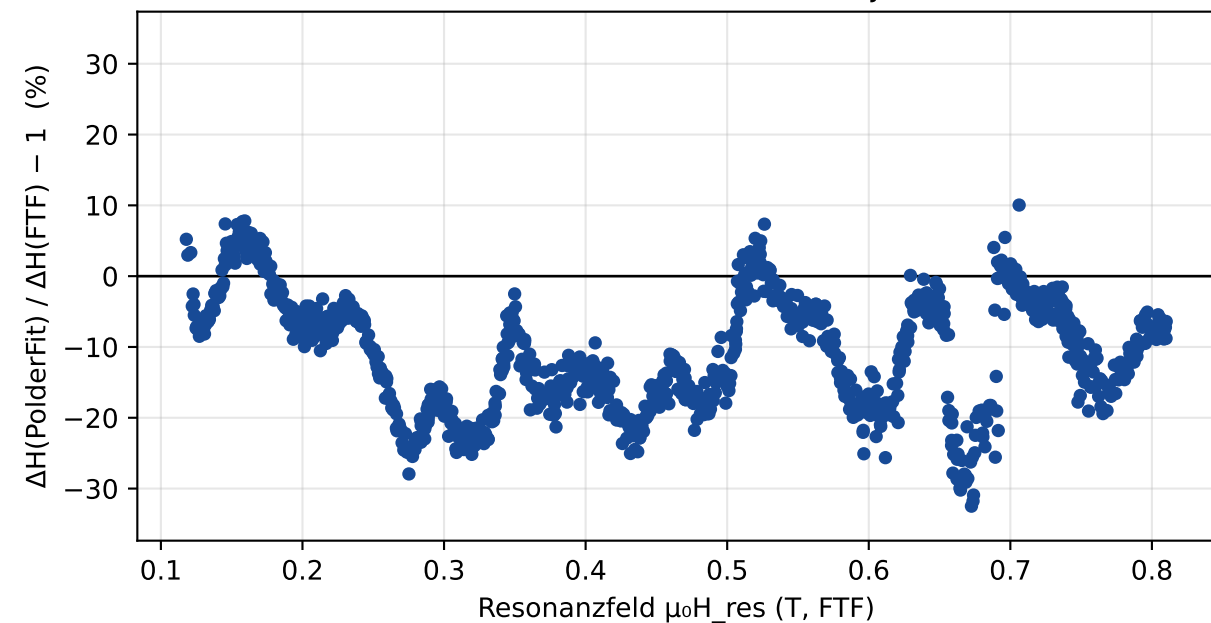
Relative Differenz Linienbreite je Feld
