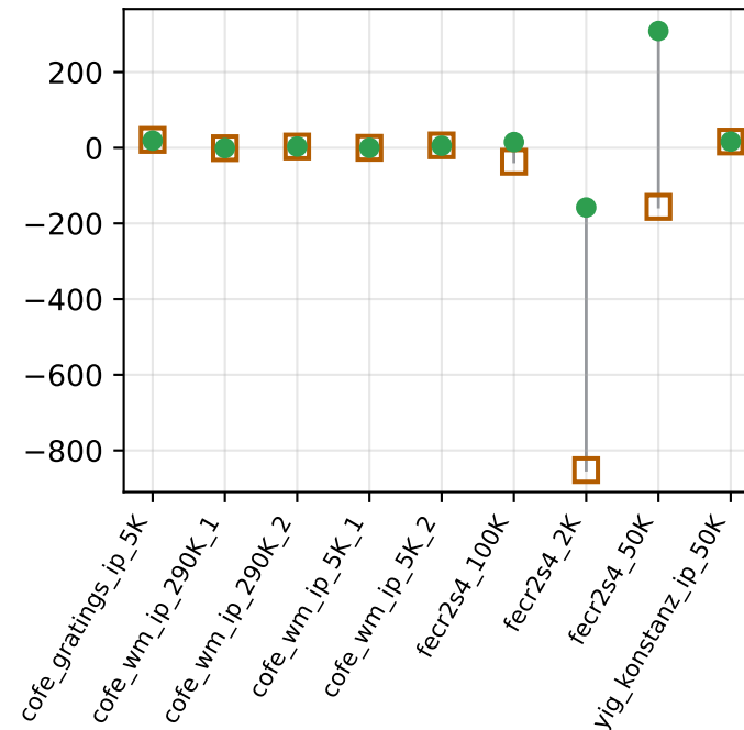
\mu_0 \Delta H_0 (mT)
