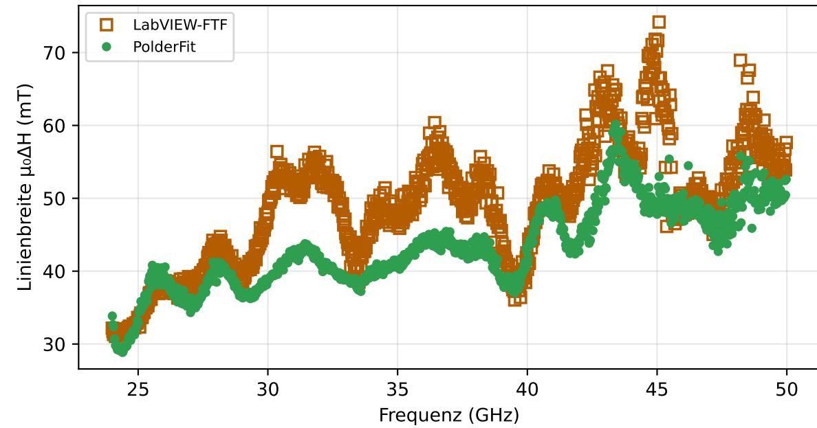
Differenz Linienbreite je Frequenz
