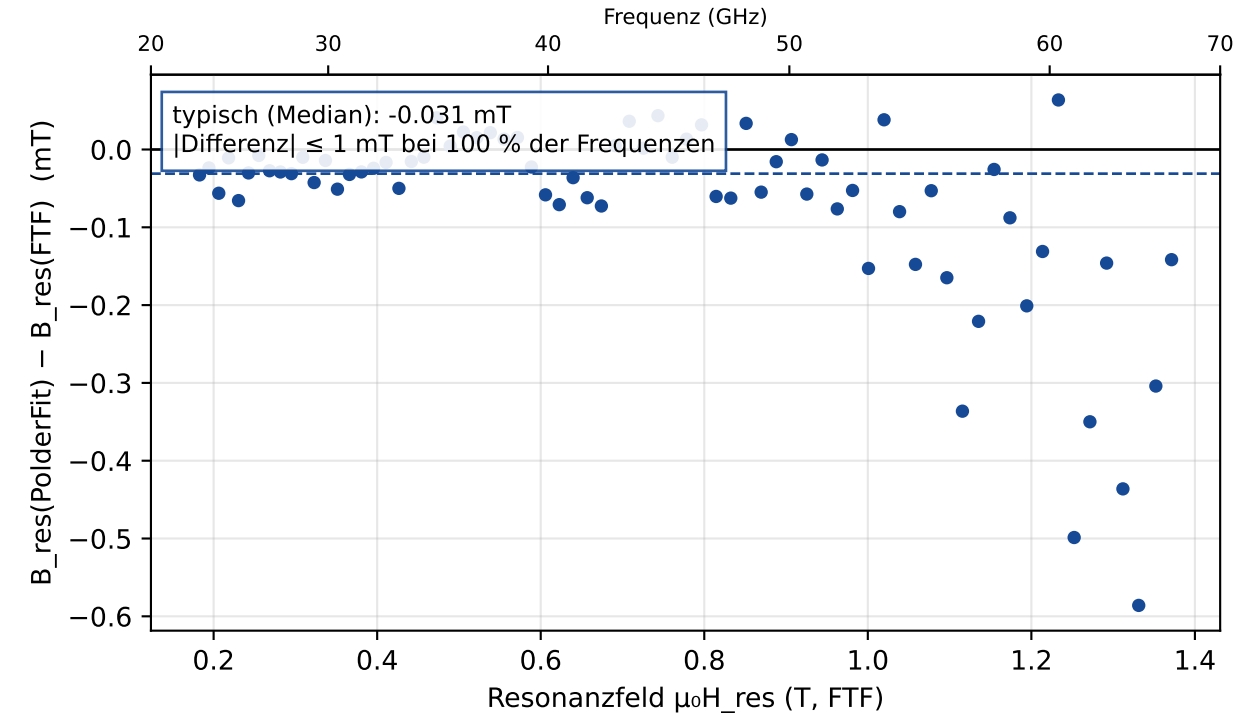
Differenz Resonanzfeld
