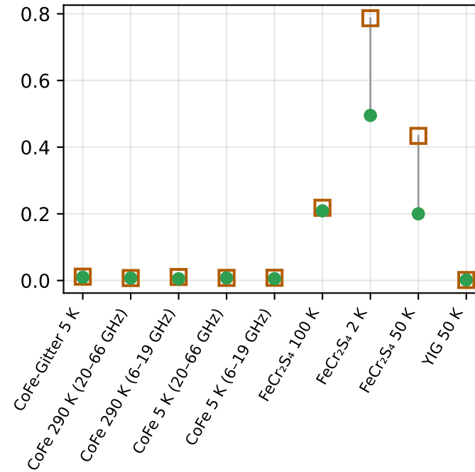
Dämpfung \alpha
