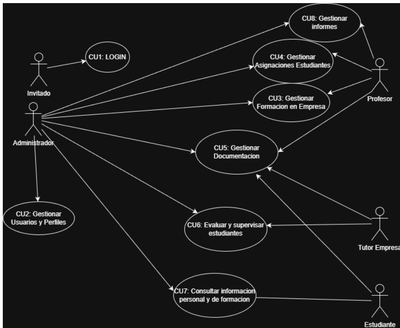
Figura 1. Primero modelo de Casos de Uso
