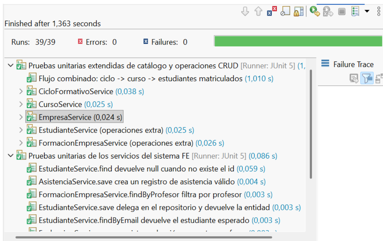
Figura 1. Ejecución de pruebas unitarias con JUnit 5 (39/39 OK)
