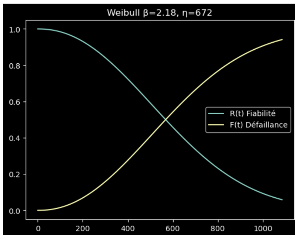
FIGURE 3.3 – Ajustement de la loi de Weibull sur les temps de défaillance (dataset IMS)
