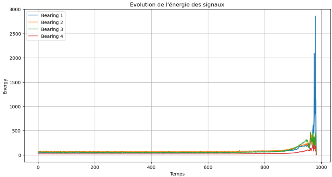
FIGURE 2.8 – Évolution de l'énergie des signaux vibratoires des roulements IMS
