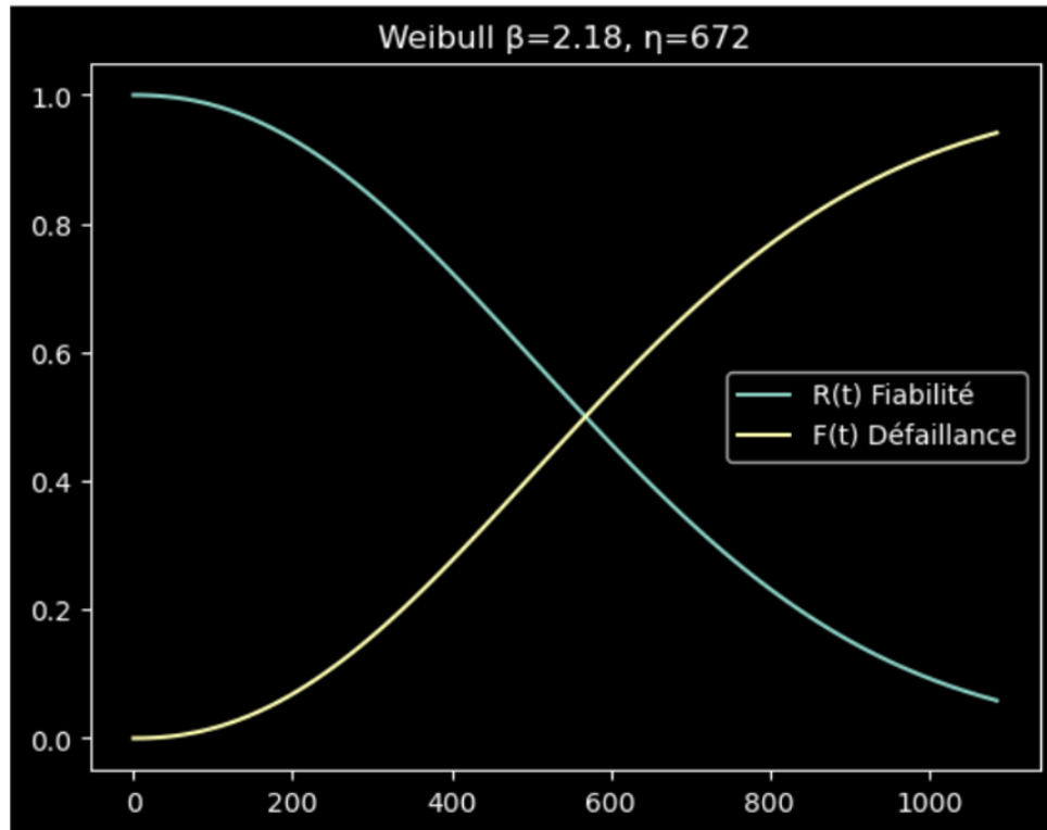
FIGURE 3.3 – Ajustement de la loi de Weibull sur les temps de défaillance (IMS dataset)
