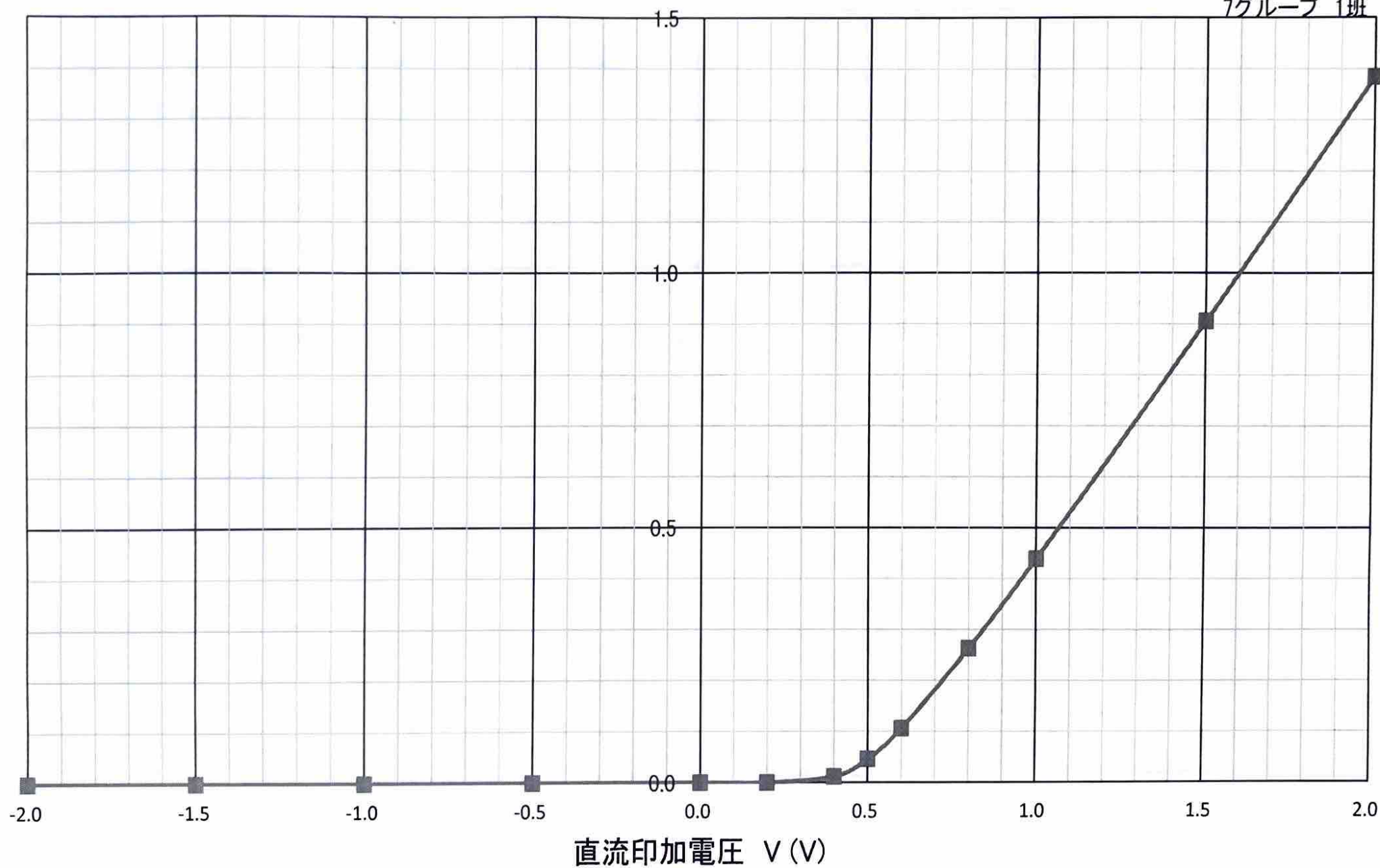
図4.1 実験1. 手動計測:シリコン・ダイオード(1S1588)の直流印加電圧-電流静特性
