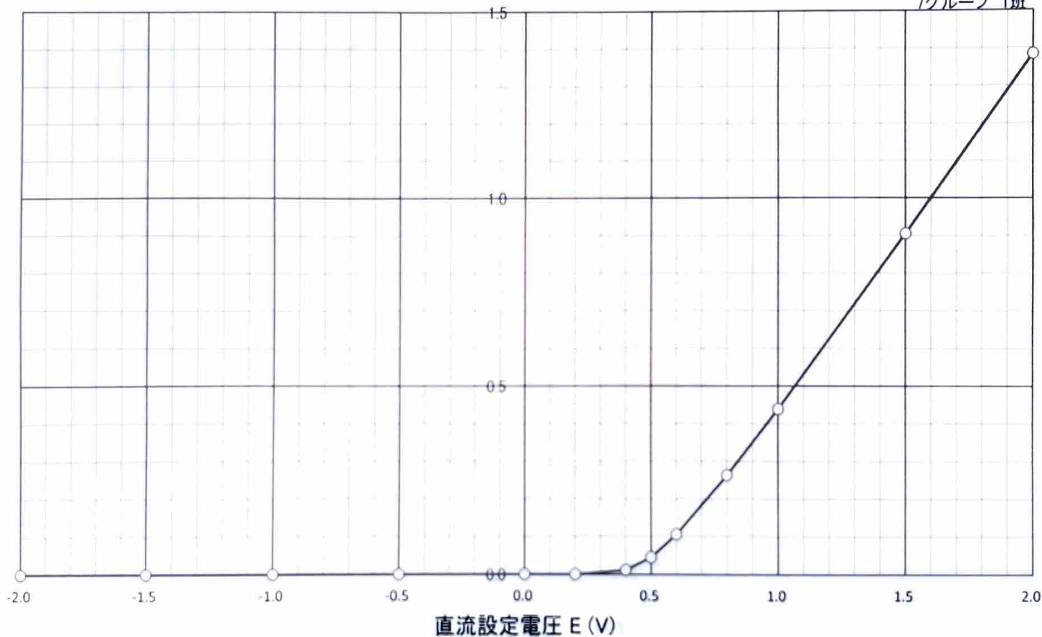
図4.2 実験3. 自動計測:シリコン・ダイオード(1S1588)の直流設定電圧-電流静特性
