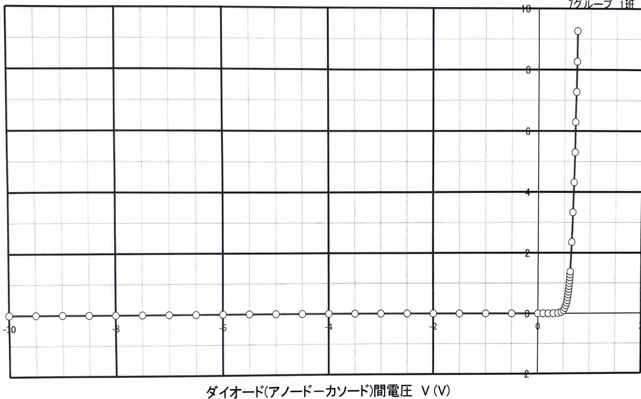
図 4.4 実験4. 自動計測_GP:シリコン・ダイオード(1S1588)の電圧-電流静特性
