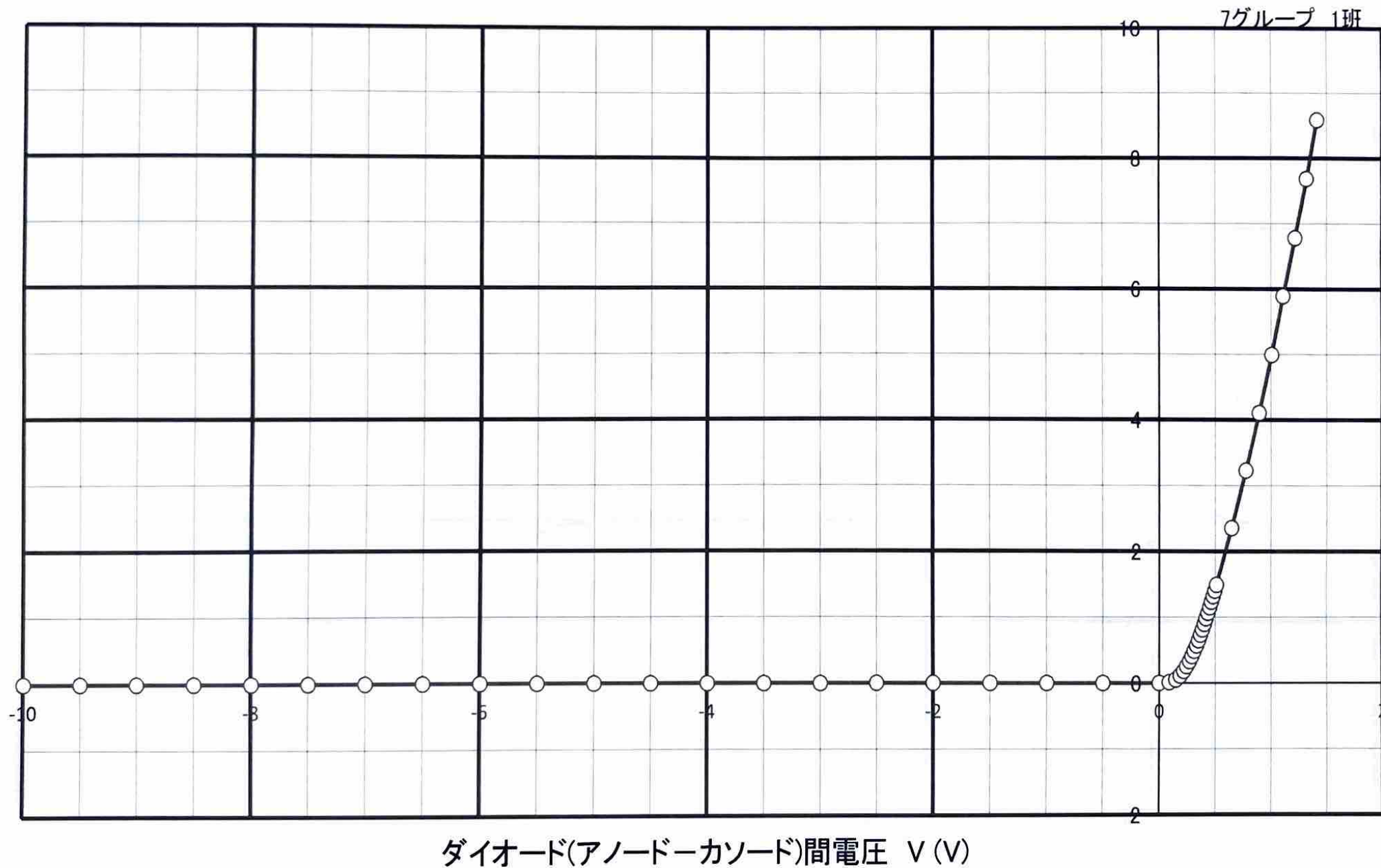
図4.5 実験4. 自動計測_GP:ゲルマニウム・ダイオード(1N60)の電圧-電流静特性
