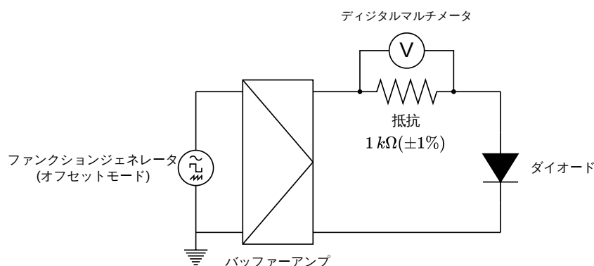
図 1 実験 1 の測定回路図
