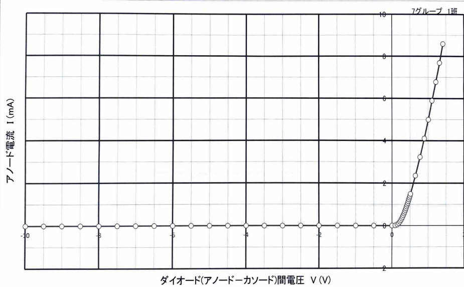
図4.5 実験4. 自動計測_GP:ゲルマニウム・ダイオード(1N60)の電圧-電流静特性
