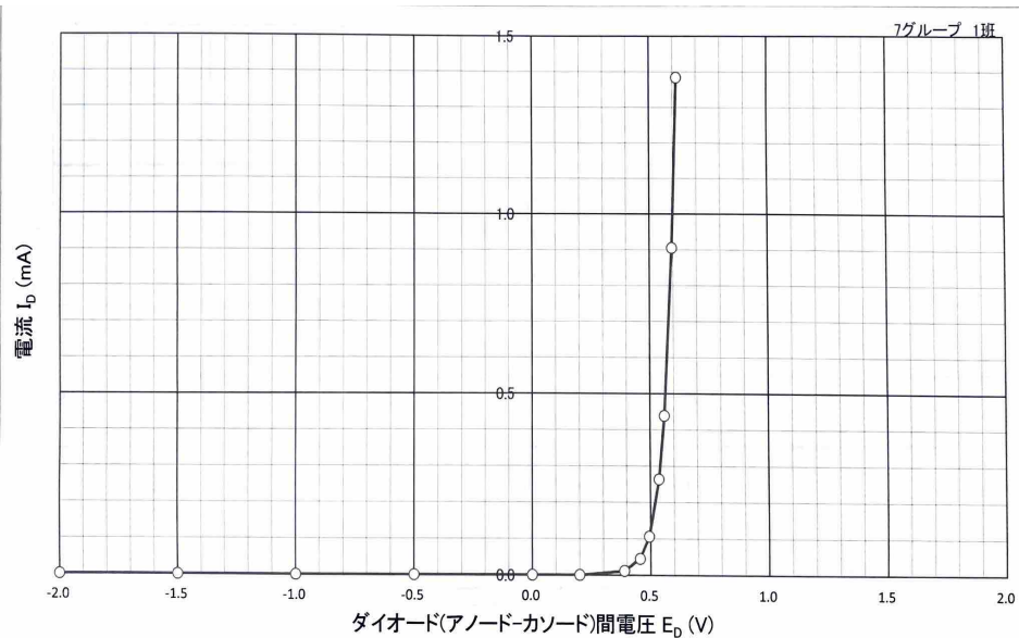
図 4.3 実験3. 自動計測:シリコン・ダイオード(1S1588)のダイオード間電圧-電流静特性
