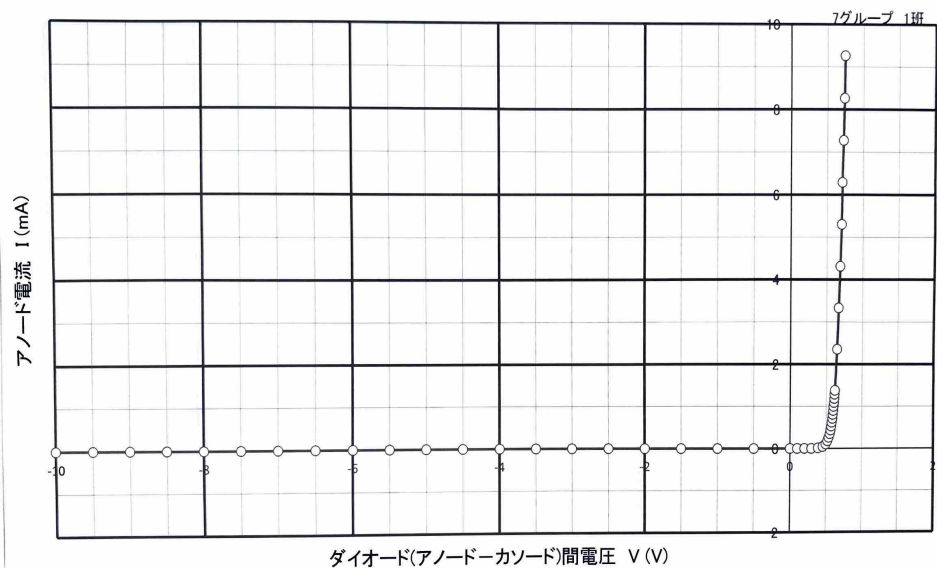
図 4.4 実験4. 自動計測_GP:シリコン・ダイオード(1S1588)の電圧-電流静特性
