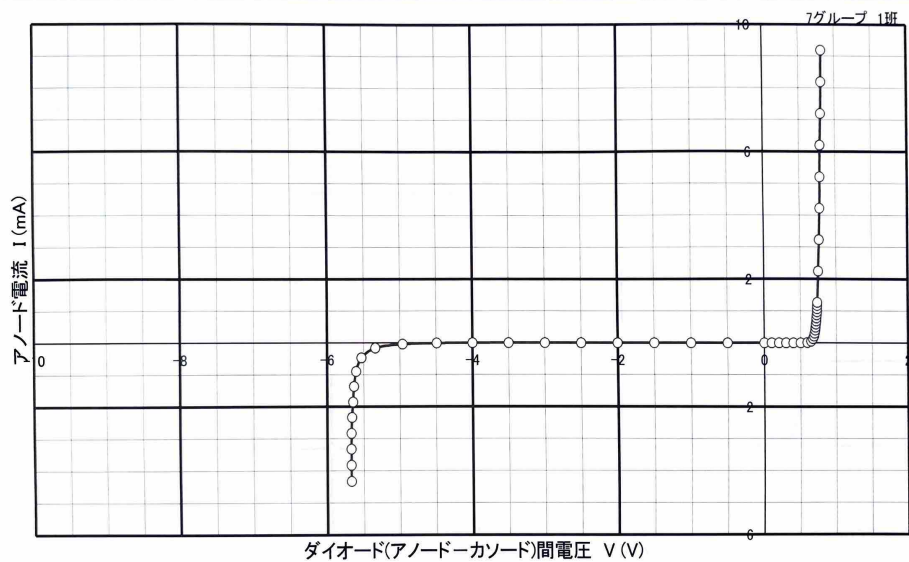
図4.6 実験4. 自動計測_GP:ツェナー・ダイオード(RD5.6E)の電圧-電流静特性
