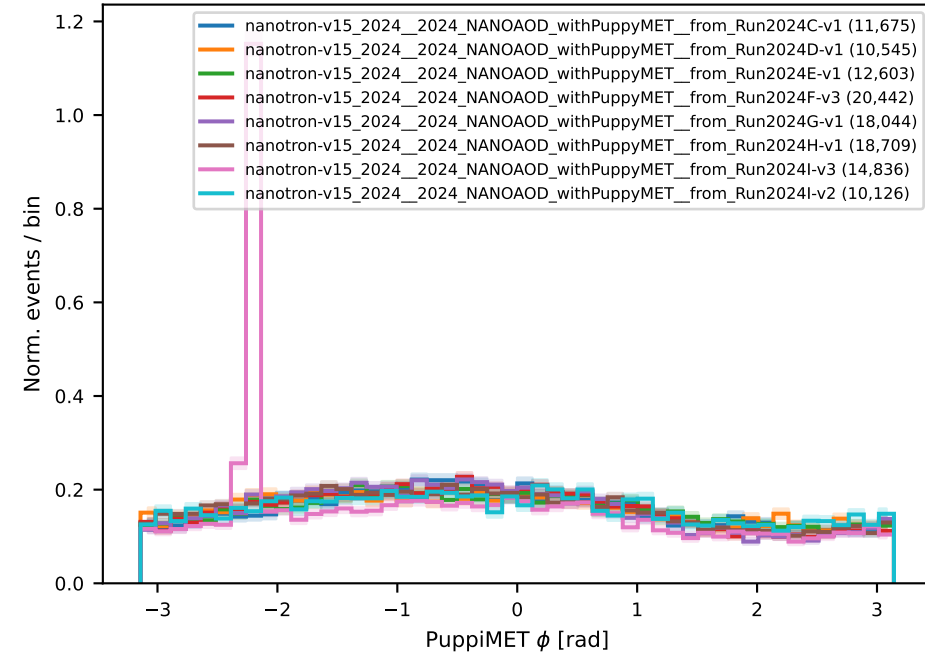
DoubleMuonLowMass1
