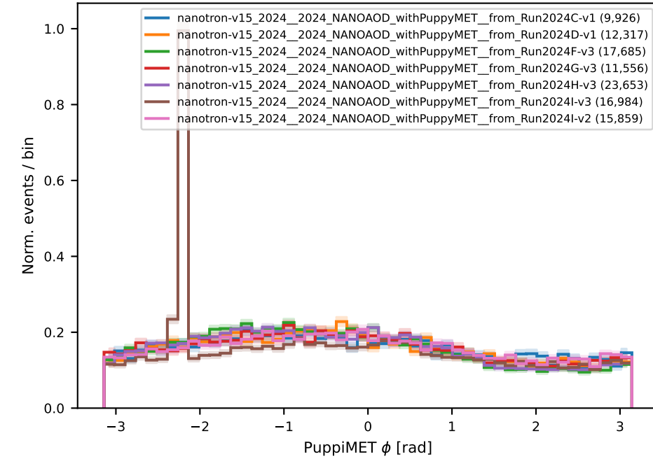
DoubleMuonLowMass0
