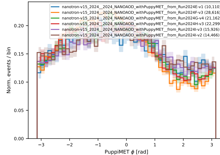
DoubleMuonLowMass7
