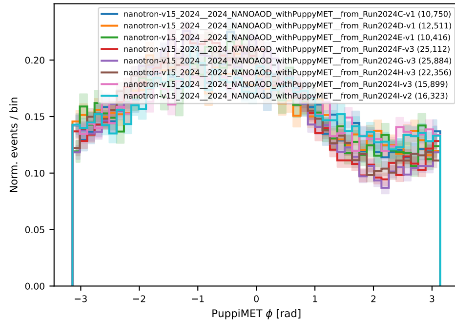
DoubleMuonLowMass4
