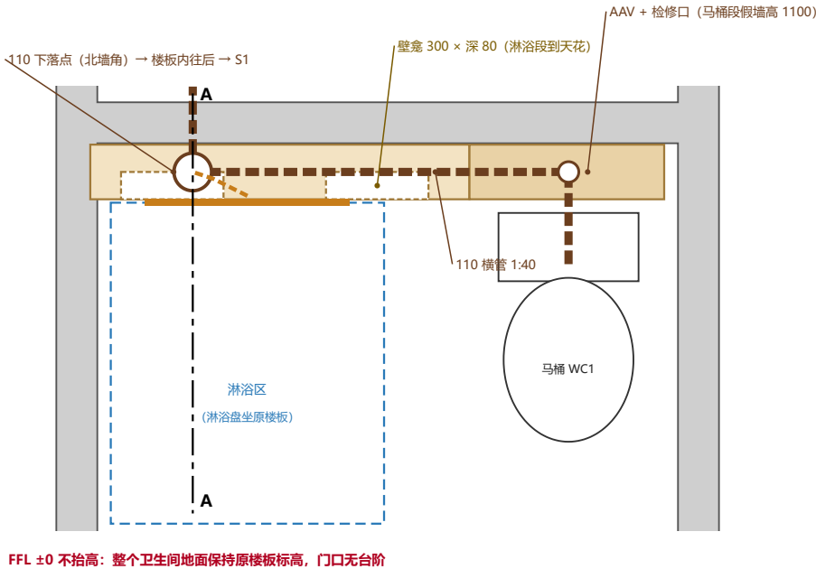
② 平面放大 Plan 1:20 (上方 = 后墙)
