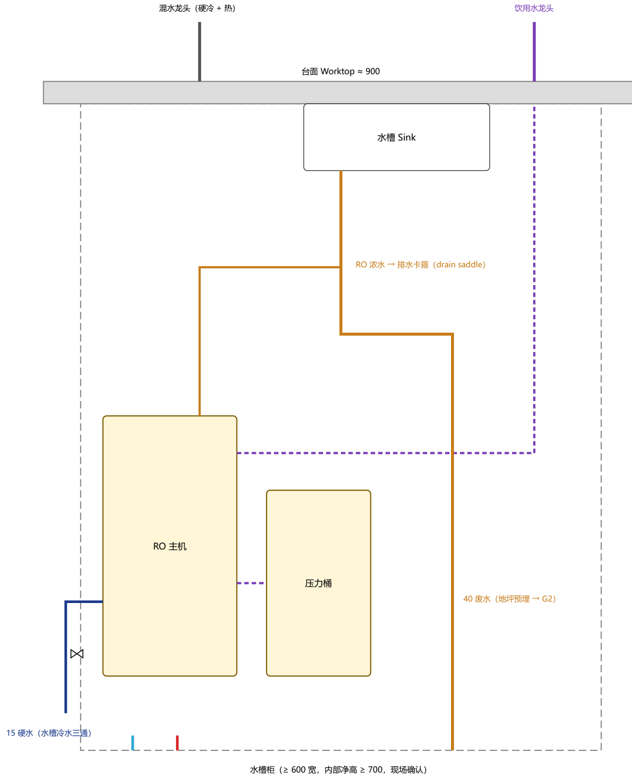
② 厨房岛台水槽下 RO 净水器 (示意)
