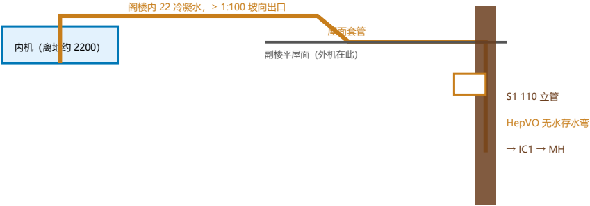
冷凝水怎么排出去 (示意剖面)
