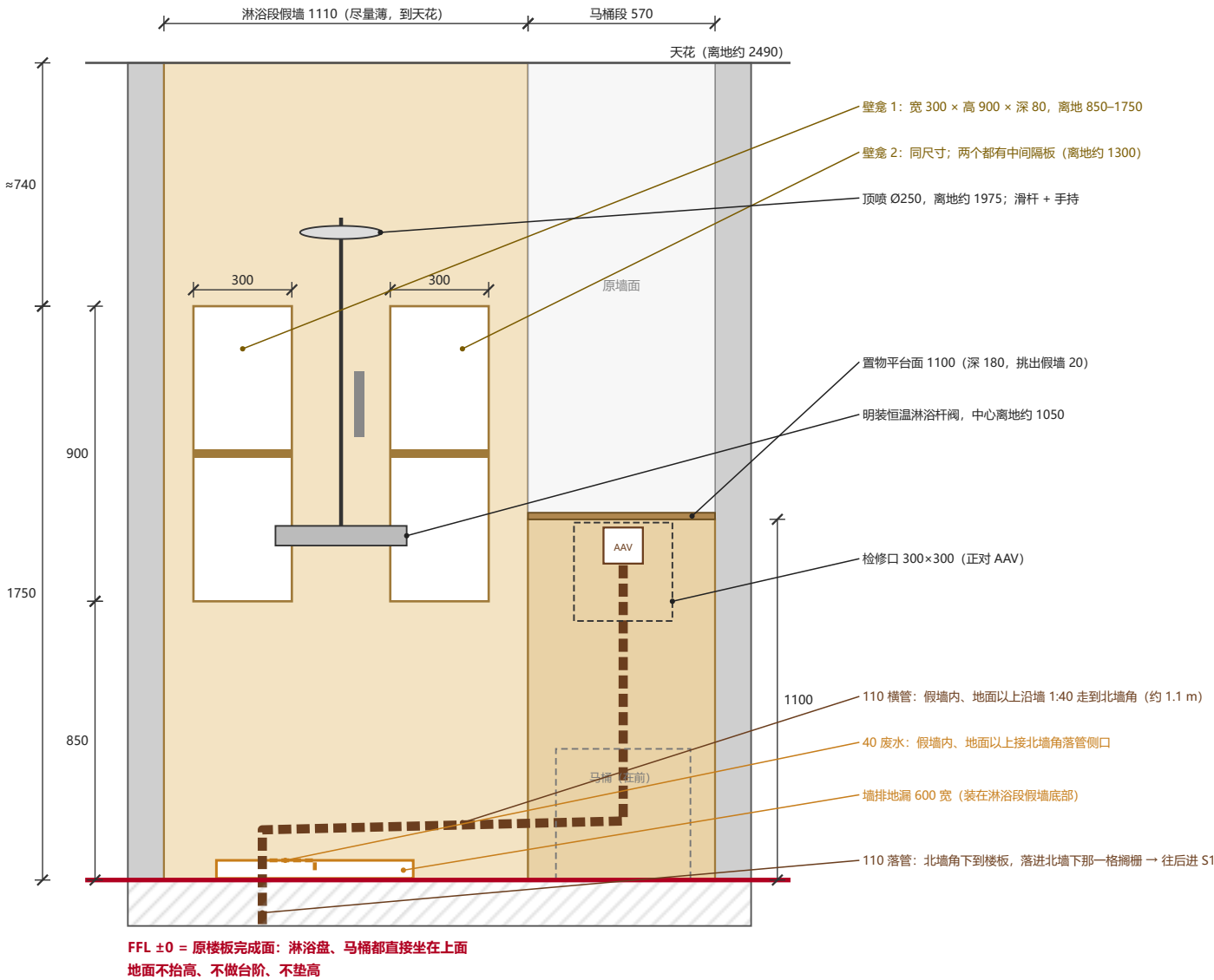
① 后墙立面 Elevation (站在卫生间里面朝后墙看) 1:20
