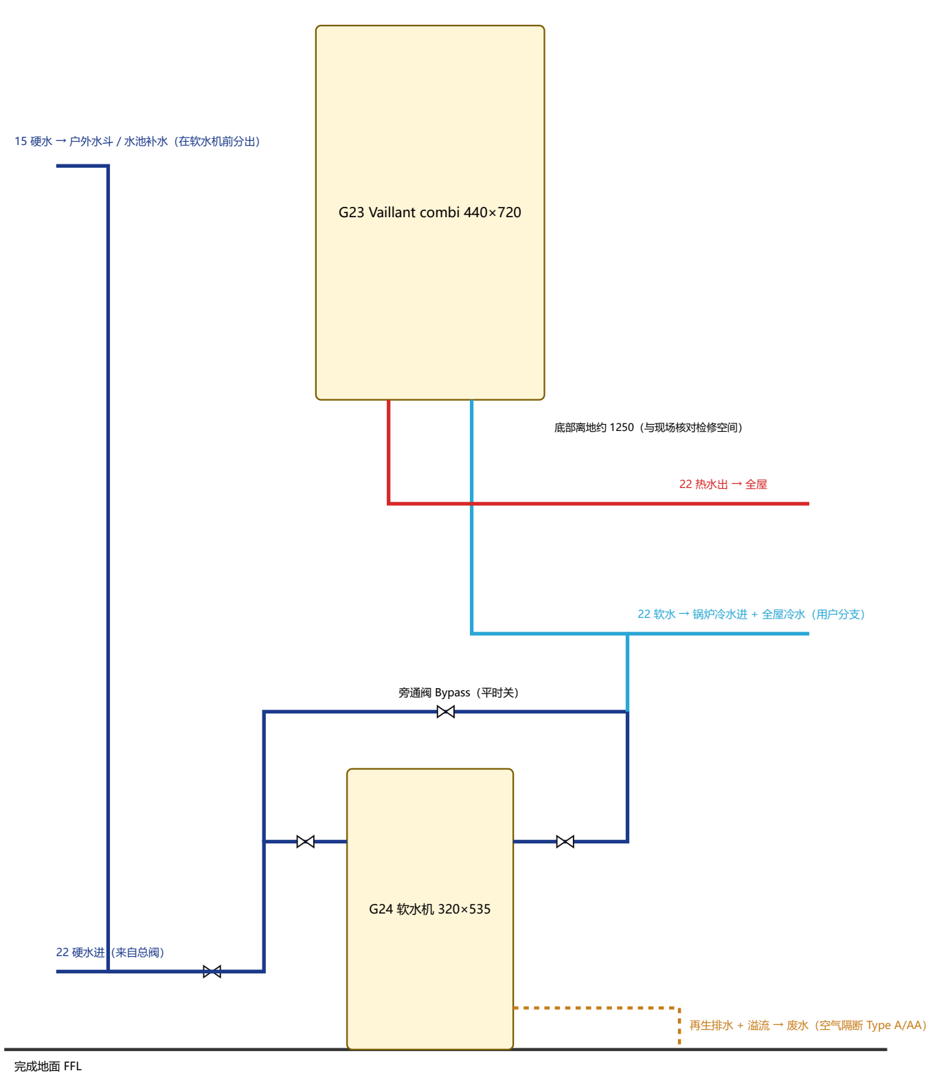
① 锅炉 G23 + 软水机 G24 立面 (厨房后墙, 示意 1:10)
