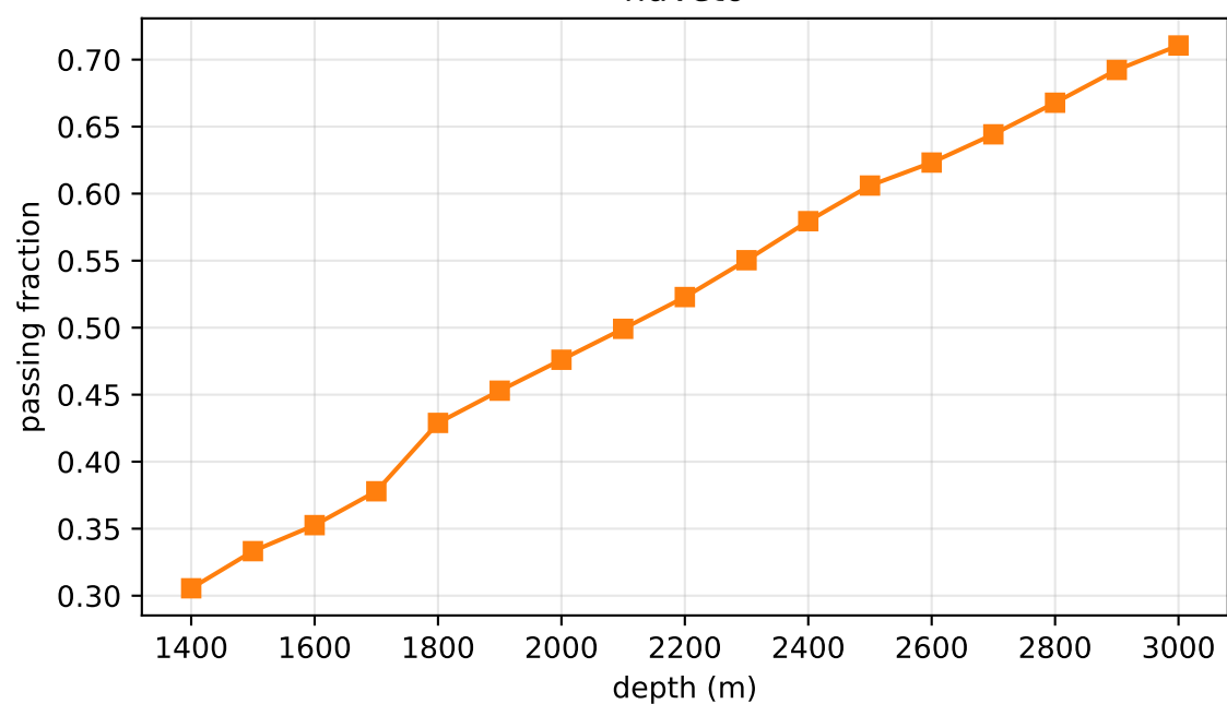
nuVeto
