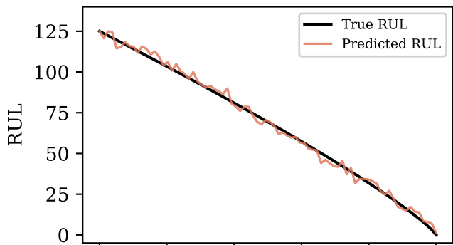
FD001 (1 op. / 1 fault)
