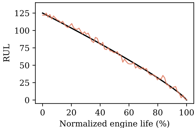
FD003 (1 op. / 2 faults)
