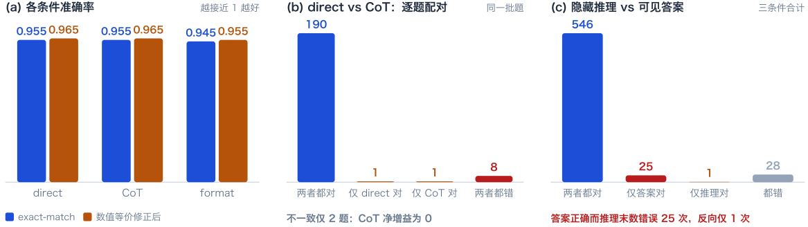
GSM8K 上的思维链消融 (n=200 题 × 3 条件, 模型 global:deepseek-v4.1-flash)
