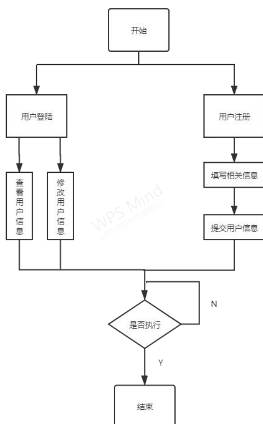
图 2.2.用户信息管理业务流程图
