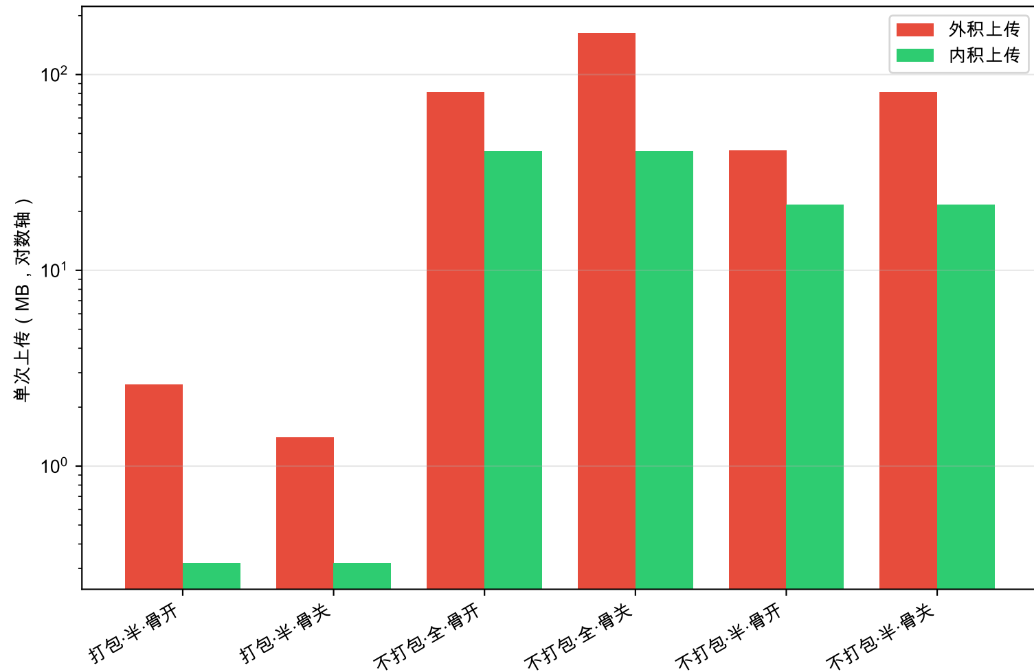
(b) 外积 vs 内积 单次上传量
