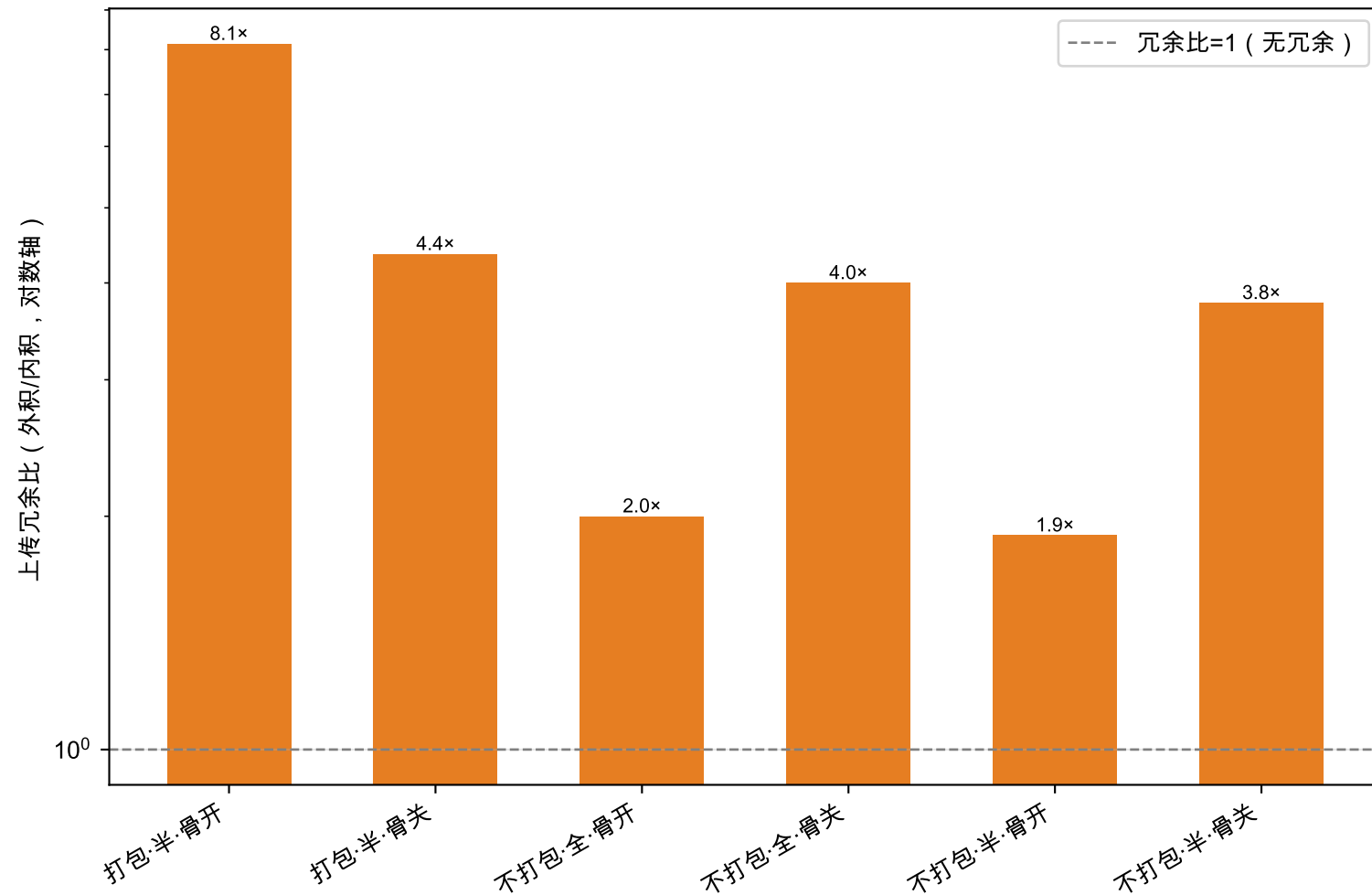
(a) 上传冗余比
