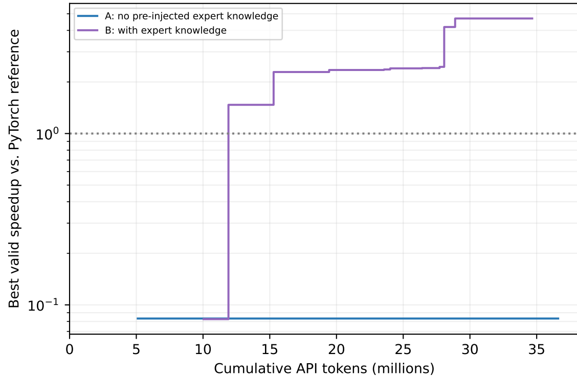
sparse_attention
