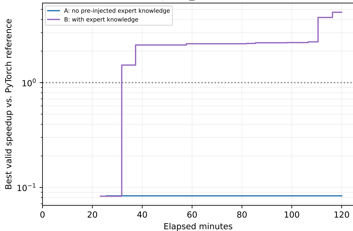
sparse_attention
