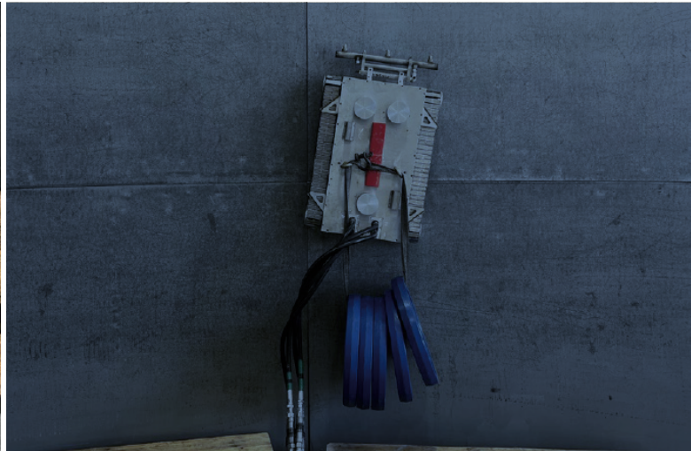
탱크 내외벽 부착형 이동 로봇 (Working robot the inner and outer walls of the storage tank)
