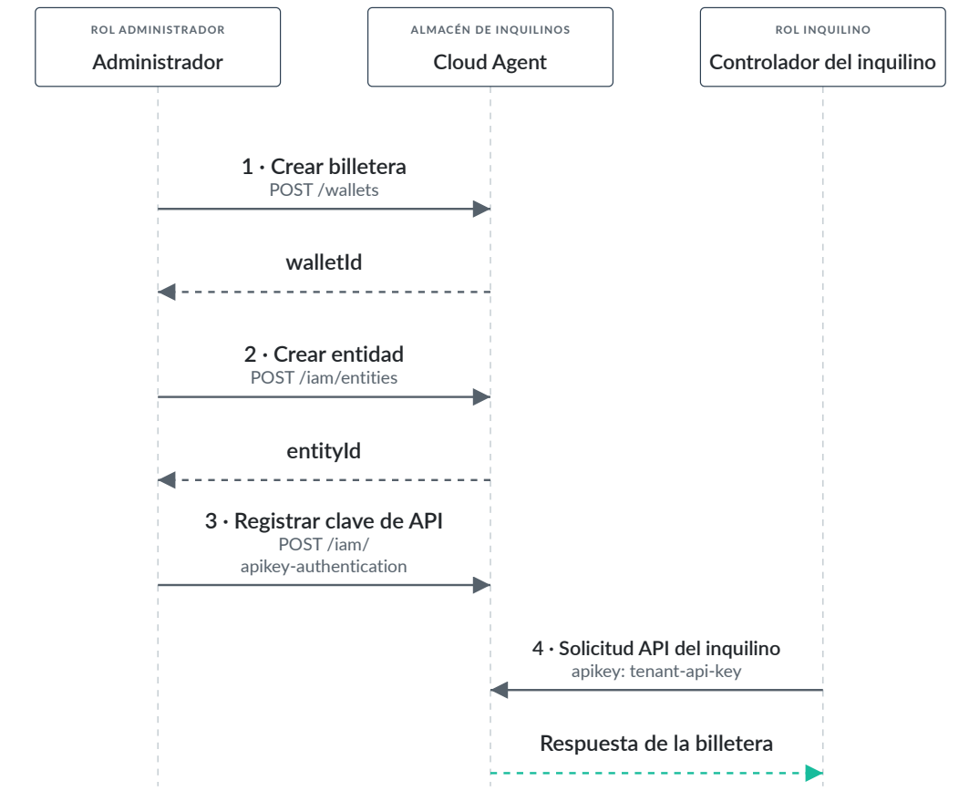
Figura 3: Con API_KEY_AUTO_PROVISIONING=false , el administrador crea la billetera, la entidad y la clave de API. La clave de API del inquilino selecciona la billetera asignada a la entidad.
