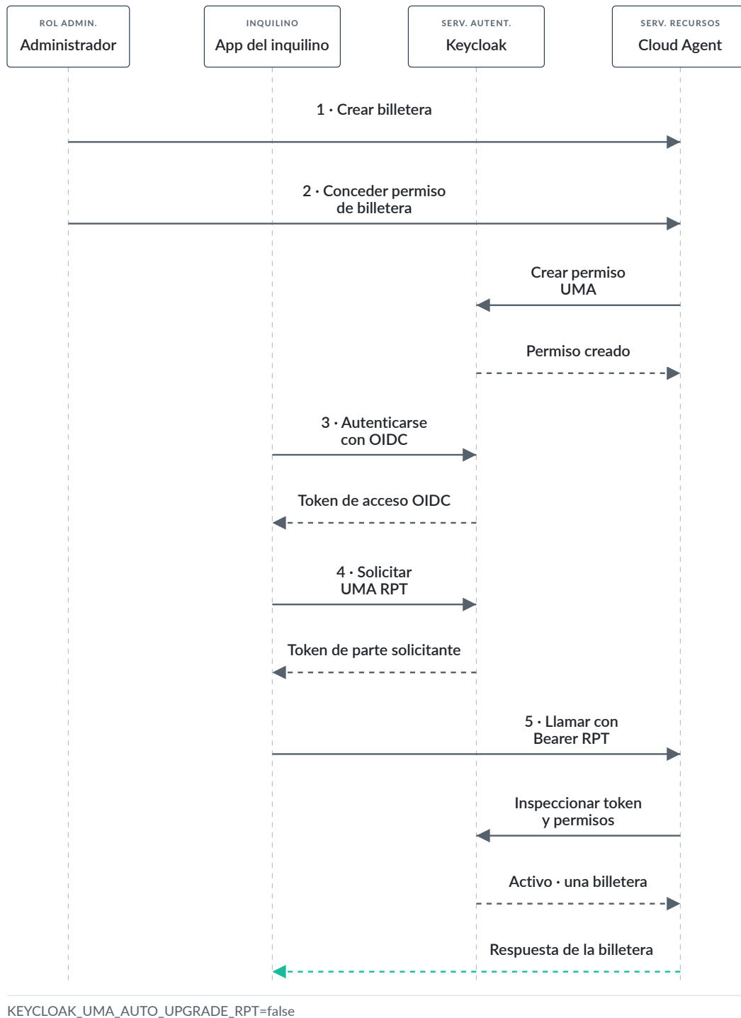
Figura 4: El administrador concede a un sujeto Keycloak acceso a una billetera de Cloud Agent. Con la conversión automática a RPT deshabilitada, el controlador del inquilino obtiene el RPT. El agente acepta una billetera autorizada por solicitud del inquilino.
