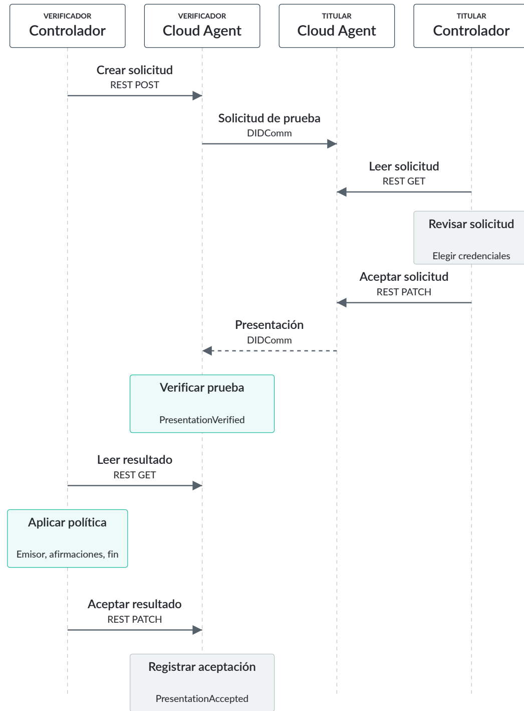
Figura 1: El verificador proporciona la vinculación de la solicitud para el formato elegido: challenge y domain para JWT o SD-JWT con vinculación de clave, o un nonce de AnonCreds. El controlador del titular selecciona credenciales y llama a request-accept. Después de PresentationVerified, el controlador del verificador comprueba su política y llama a presentation-accept solo si supera las comprobaciones. Un rechazo por política detiene la acción de la aplicación. Este diagrama sigue el flujo correcto y omite respuestas REST.
