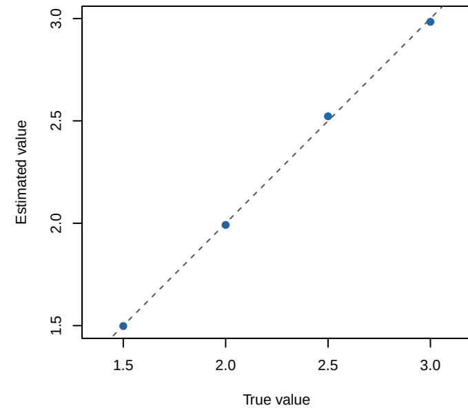
adjoint pmmr
