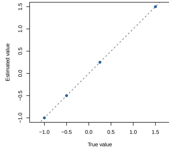
adjoint pmmr
