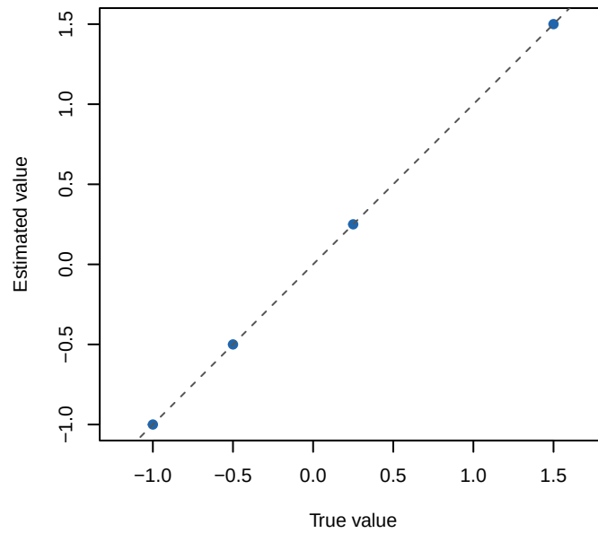
adjoint landweber
