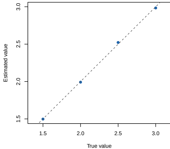
adjoint sieve_md
