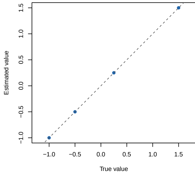
adjoint sieve_md
