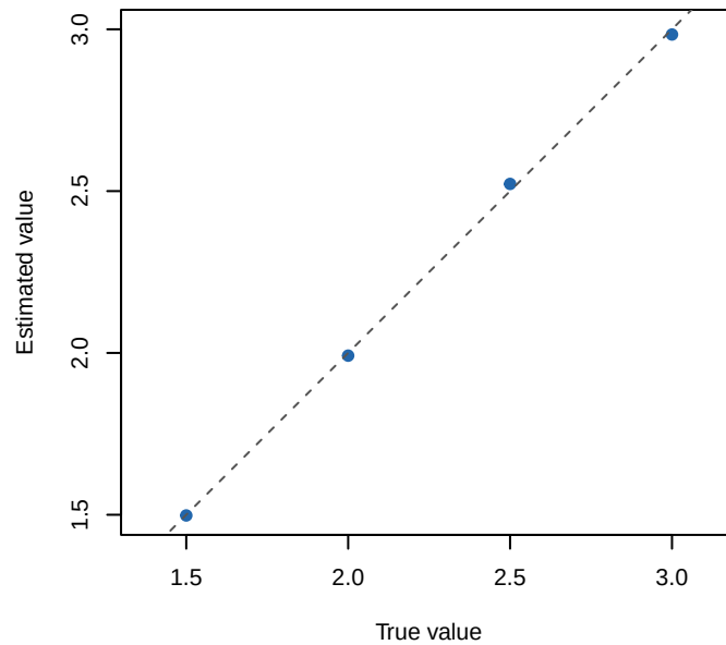
adjoint landweber
