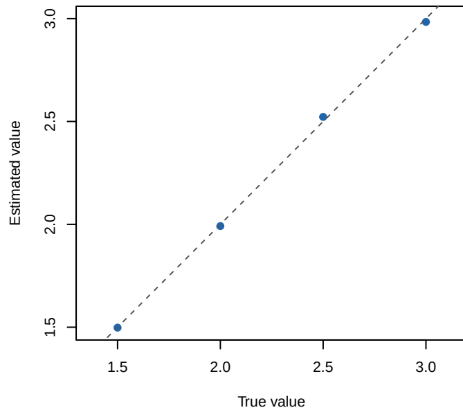
adjoint sieve_md
