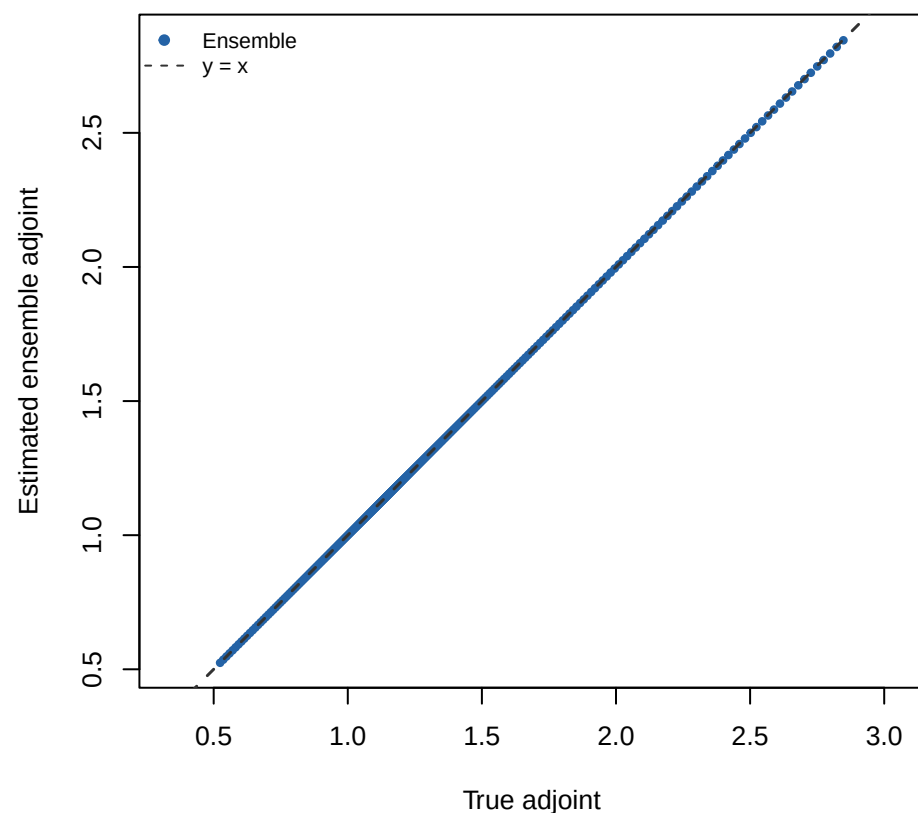
Gaussian kernel truth – adjoint
