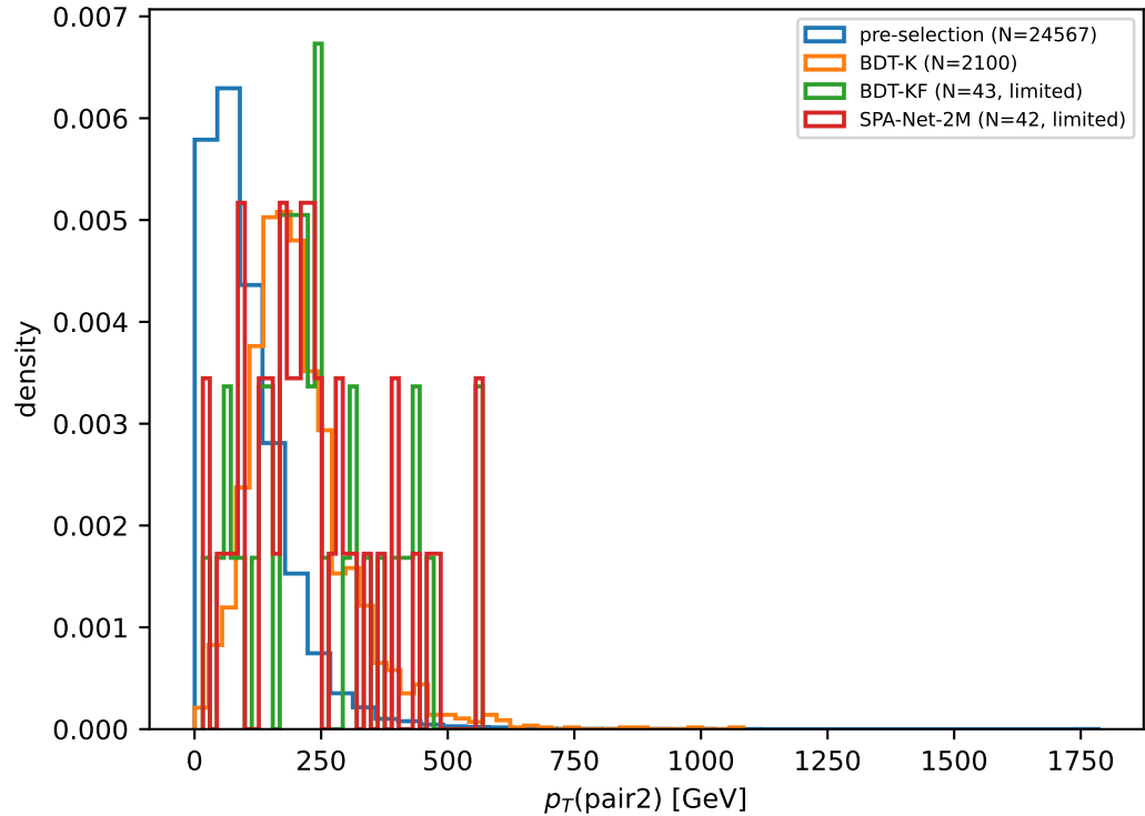
t\bar{t}b\bar{b} , \varepsilon_S=0.4 : dijet-pair p_T
