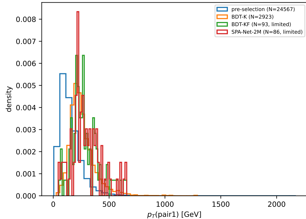
t\bar{t}b\bar{b} , \varepsilon_S=0.5 : dijet-pair p_T
