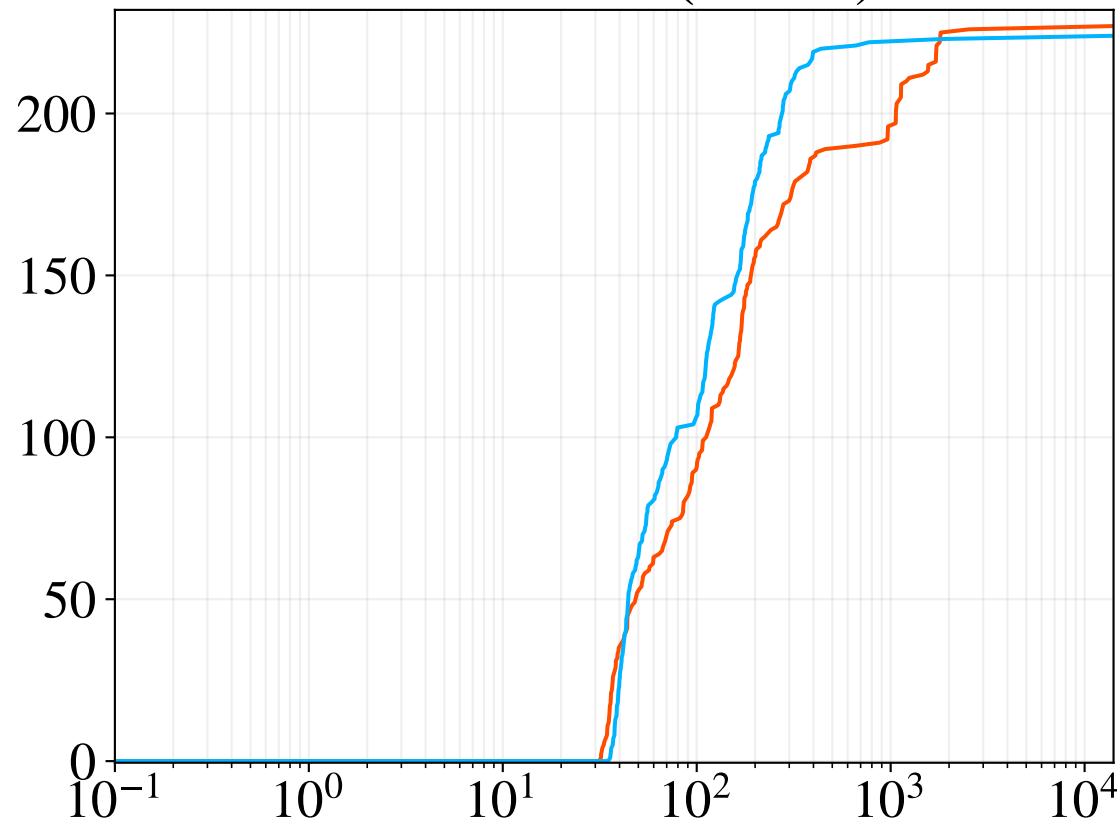
Peformance (14x28)
