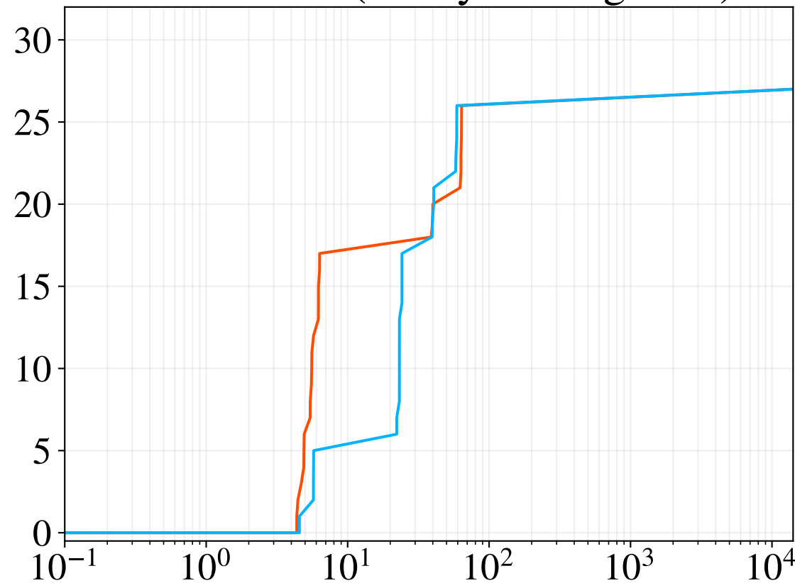
Peformance (LeakyReluSigmoid)
