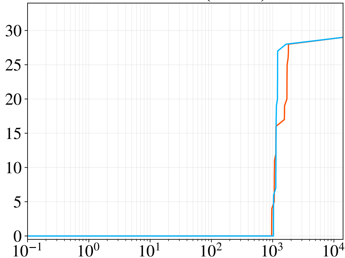
Peformance (14x28)
