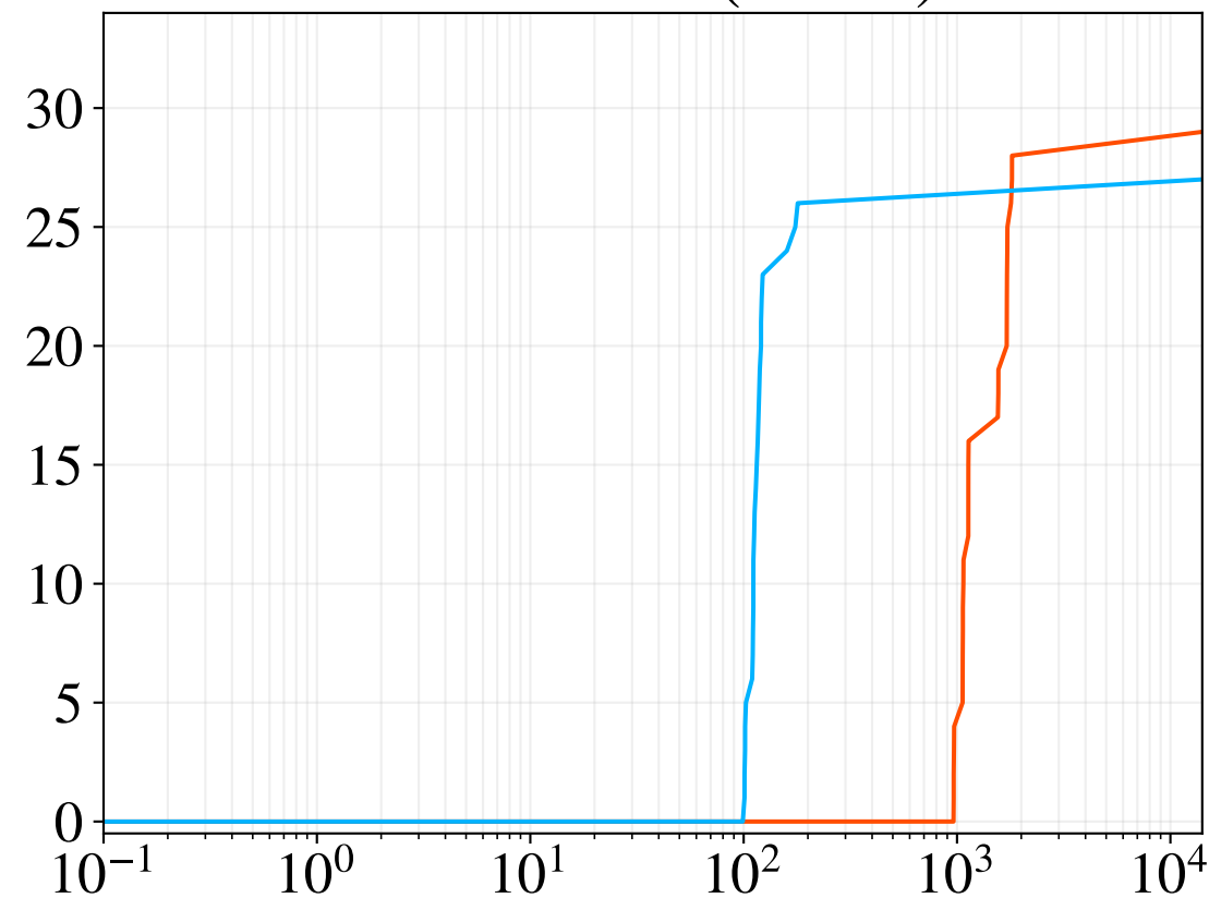
Peformance (14x28)
