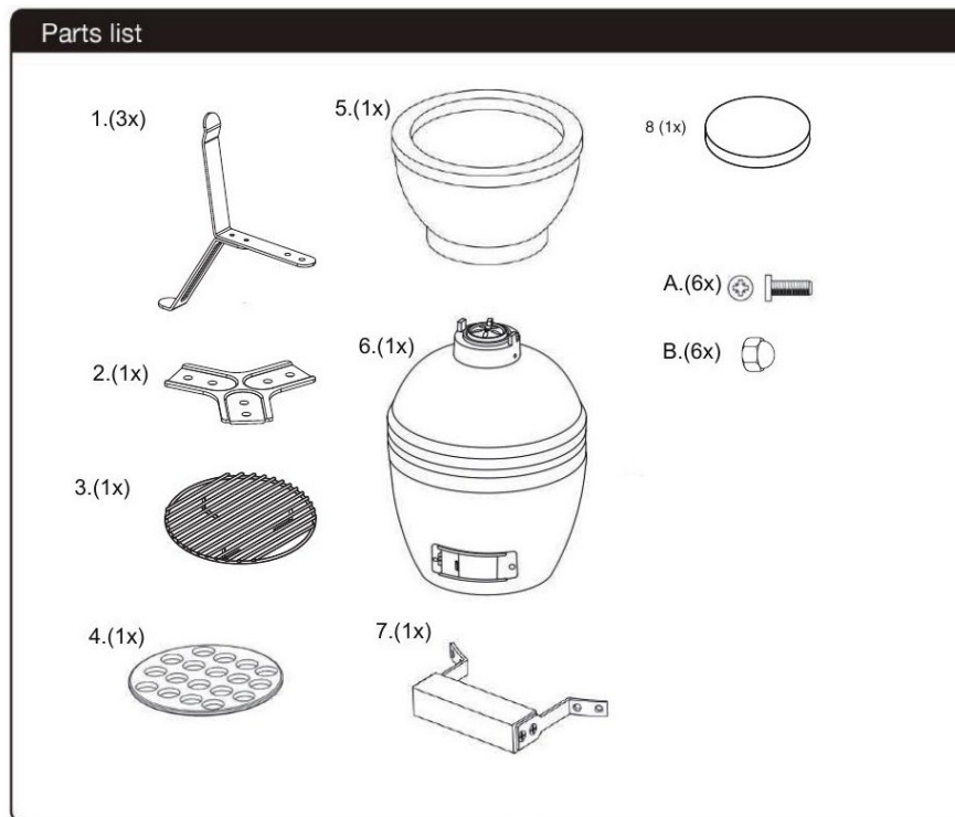
רשימת החלקים
